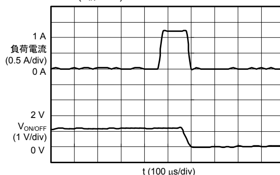
図 12 負荷短絡による間欠動作時の出力電流波形
