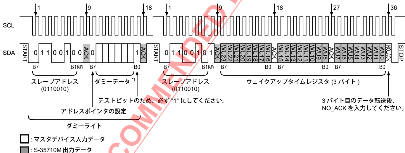
図20 ウェイクアップタイムレジスタの読み出しタイミング
