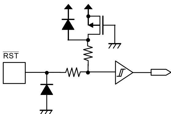
図5 RST端子
