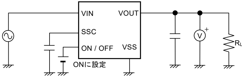
図7 測定回路5
