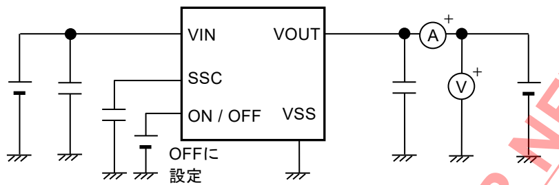
図8 測定回路6
