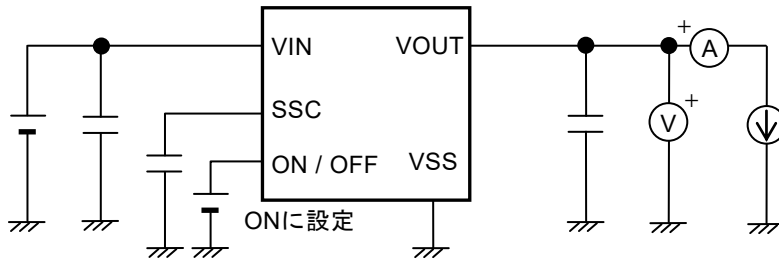
図3 測定回路1
