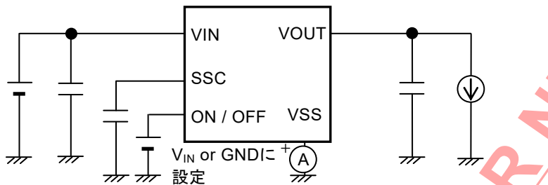
図4 測定回路2
