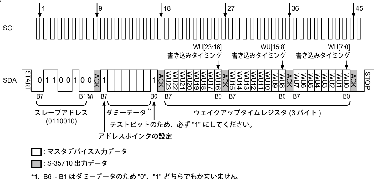
図24 ウェイクアップタイムレジスタの書き込みタイミング
