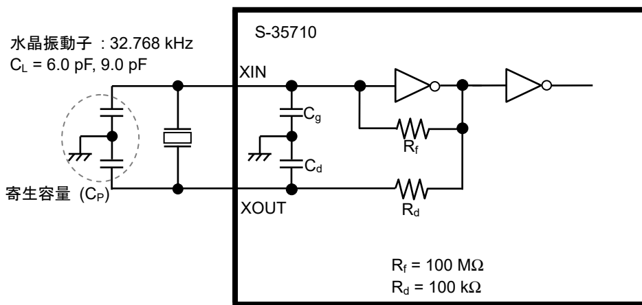
図33 水晶発振回路構成
