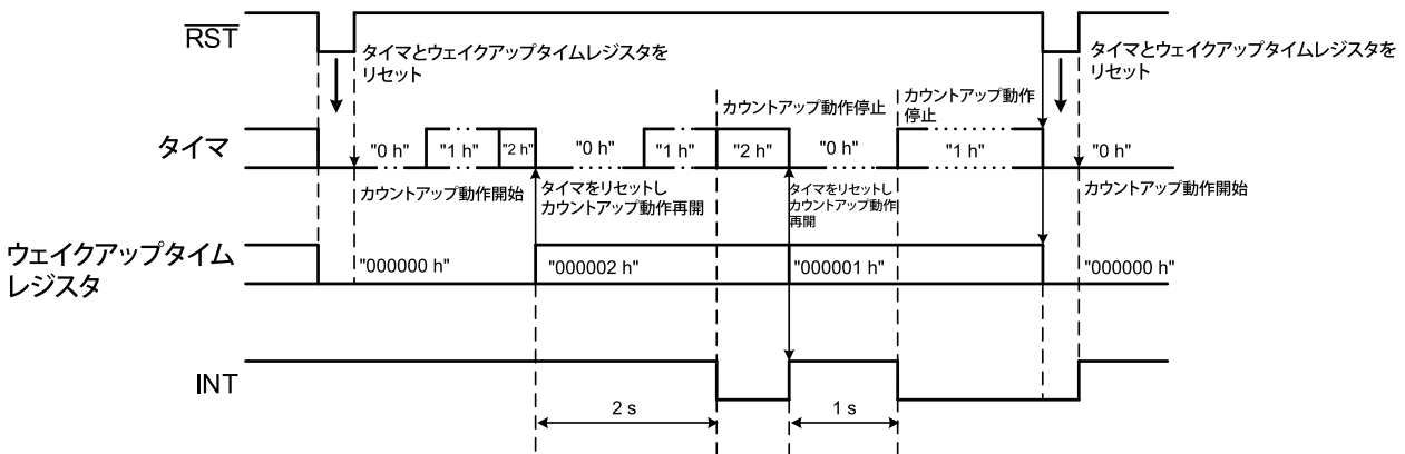
図12 ハンドシェイクタイムアウトの出力タイミング例 (S-35710C01I / Nchオープンドレイン出力)
