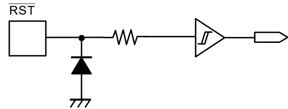
図6 \overline{\text{RST}} 端子 (S-35710C01I / プルアップ抵抗なし)
