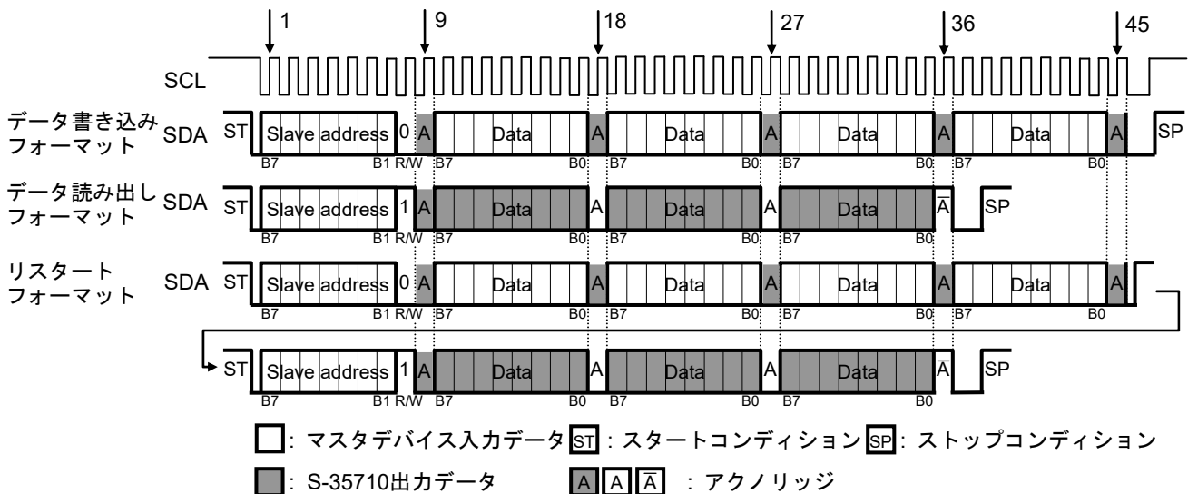
図22 シリアルインタフェースのデータ転送フォーマット
