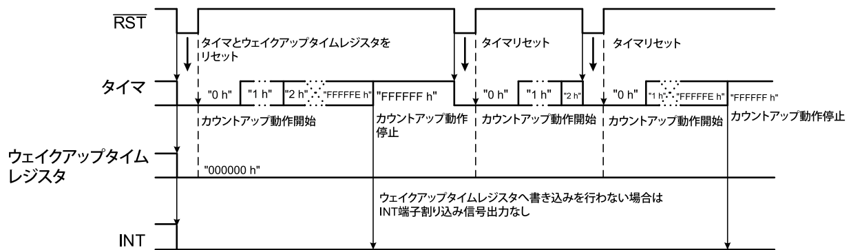
図15 ウェイクアップタイムレジスタに書き込みを行わない場合 (S-35710B011 / CMOS出力)
