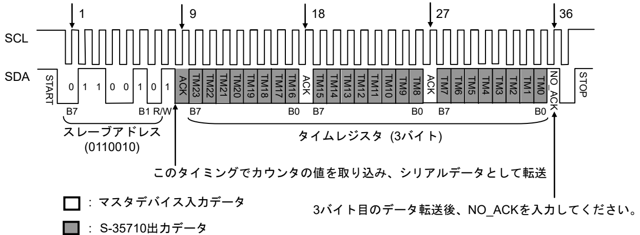
図23 タイムレジスタの読み出しタイミング
