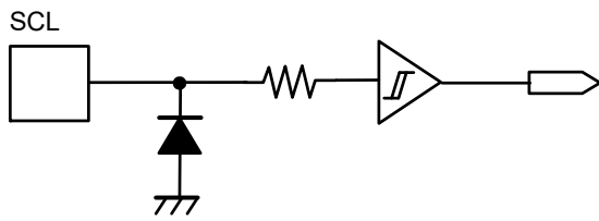
図3 SCL端子
