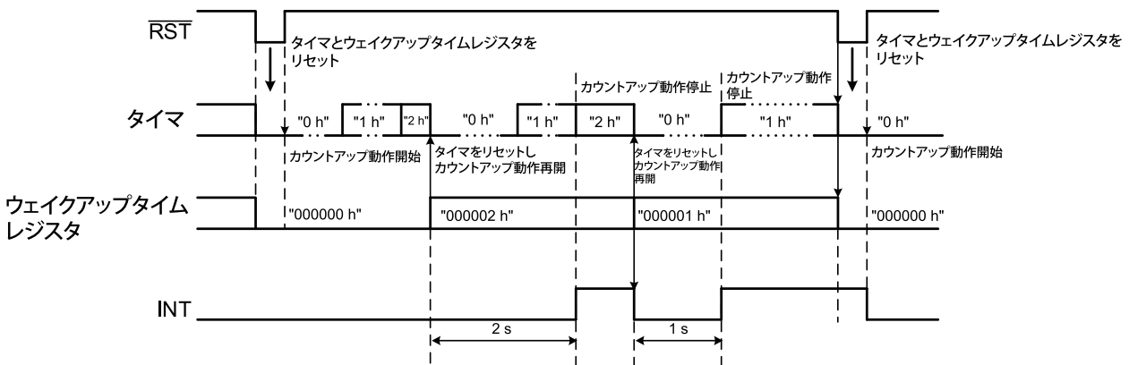
図13 ハンドシェイクタイムアウトの出力タイミング例 (S-35710B01I / CMOS出力)
