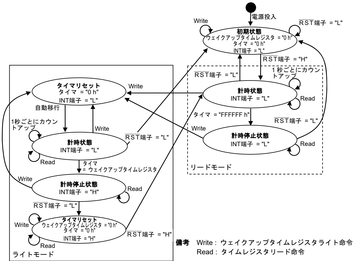
図17 ハンドシェイクタイムアウトの状態遷移図 (S-35710B011 / CMOS出力)
