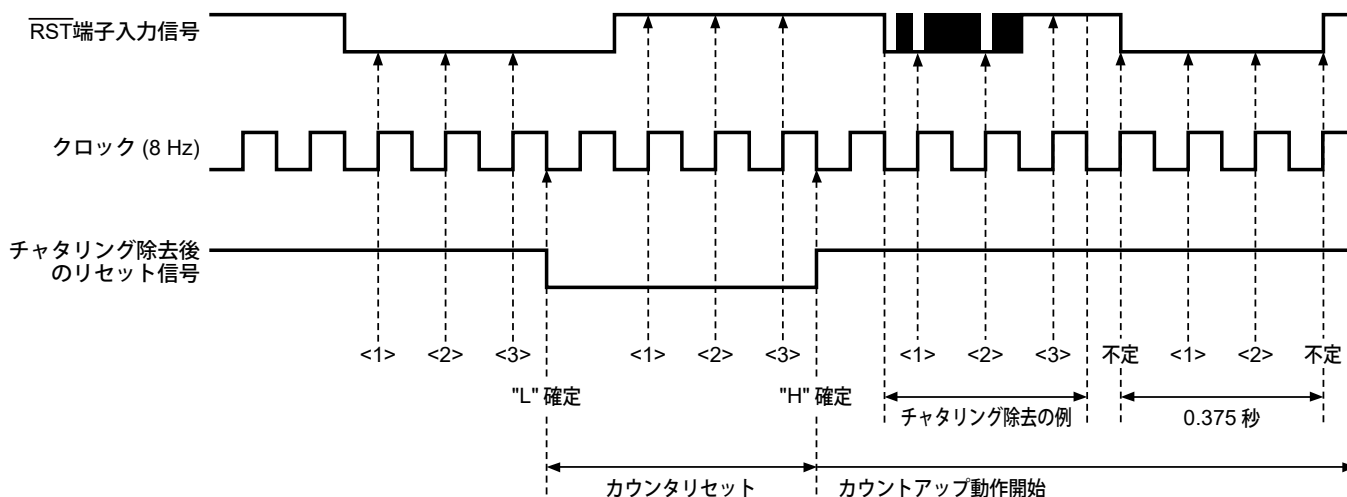
図30 チャタリング除去のタイミングチャート例
