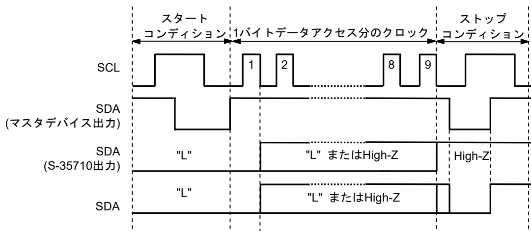
図26 SDAの解放方法
