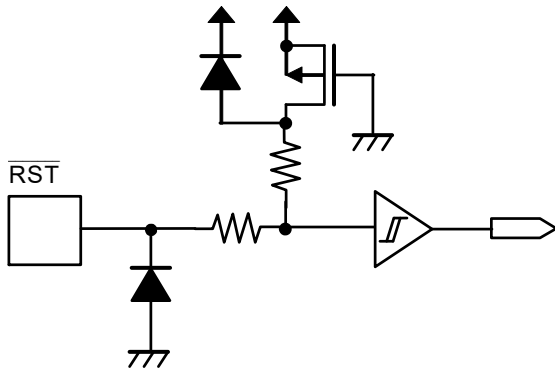
図5 \overline{\text{RST}} 端子 (S-35710B01I / プルアップ抵抗あり)
