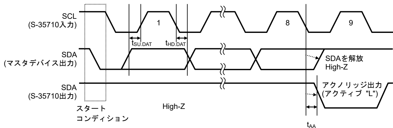
図21 アクノリッジ出力タイミング
