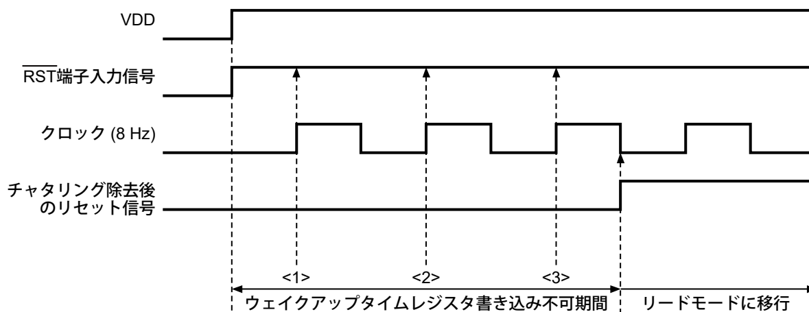
図31 電源投入時のタイミングチャート
