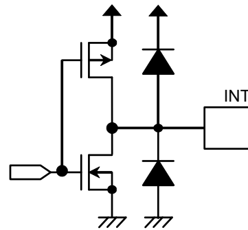
図8 INT端子 (S-35710B01I / CMOS出力)
