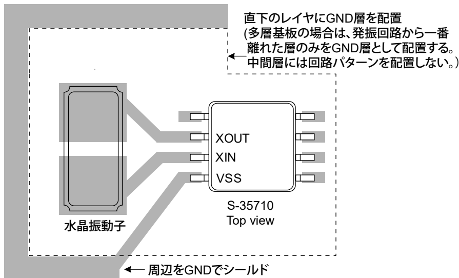
図34 接続パターン図の推奨例
