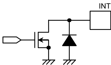
図7 INT端子 (S-35710C01I / Nchオープンドレイン出力)
