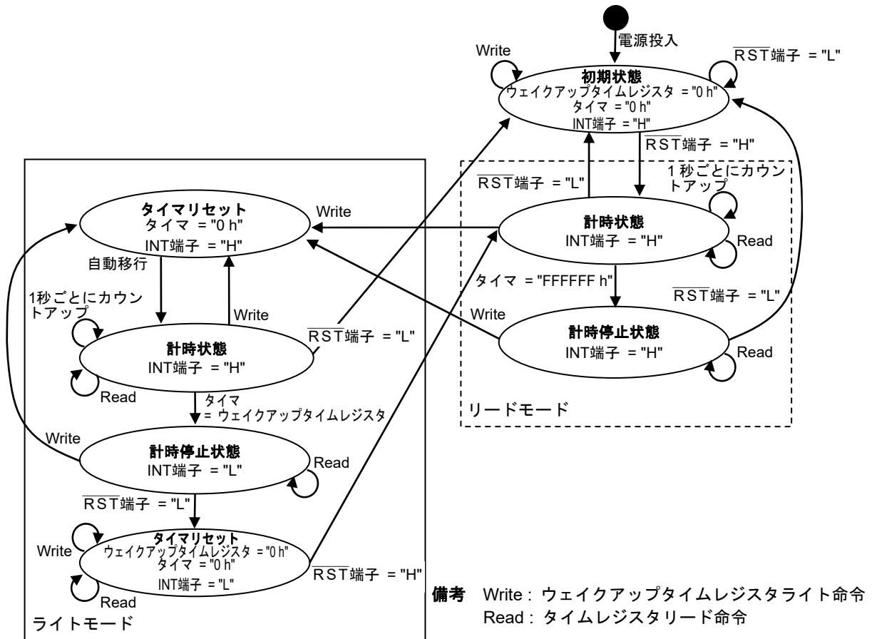
図16 ハンドシェイクタイムアウトの状態遷移図 (S-35710C01I / Nchオープンドレイン出力)
