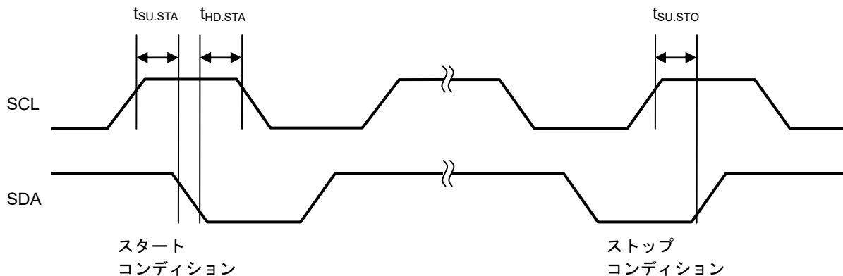
図20 スタート / ストップコンディション
