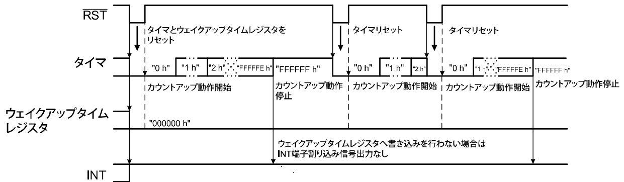
図14 ウェイクアップタイムレジスタに書き込みを行わない場合 (S-35710C011 / Nchオープンドレイン出力)
