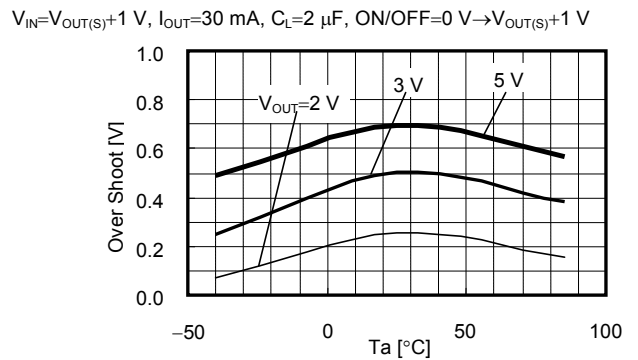
ON-OFF 投入オーバーシュートの温度依存性
