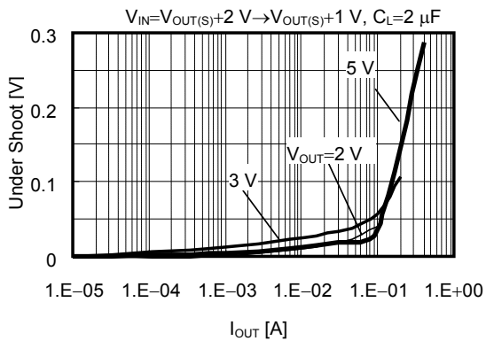
電源変動アンダーシュートの負荷依存性
