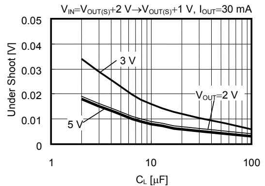
電源変動アンダーシュートの C_L 依存性
