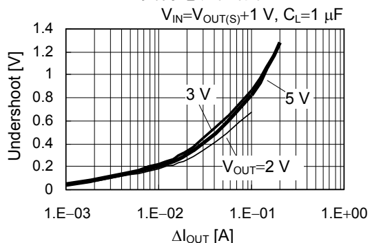
アンダーシュートの負荷電流依存性
