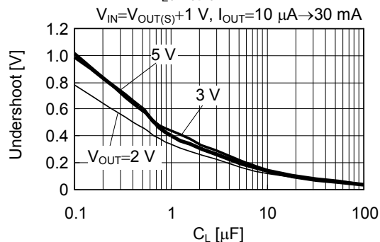
アンダーシュートのC L 依存性
