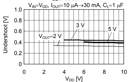
アンダーシュートのV DD 依存性
