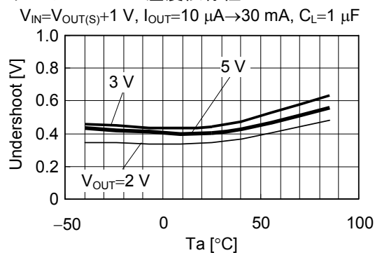
アンダーシュートの温度依存性
