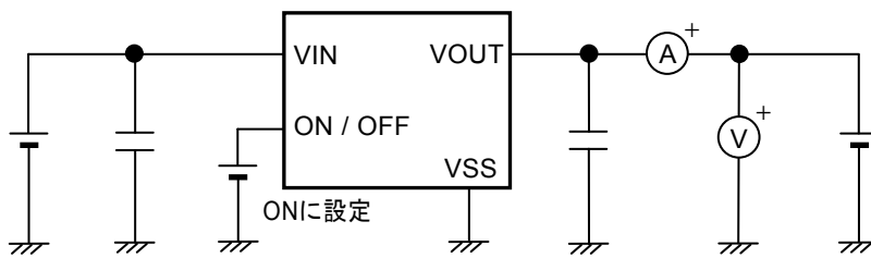
図15 測定回路6
