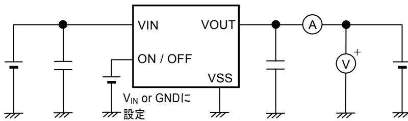
図12 測定回路3
