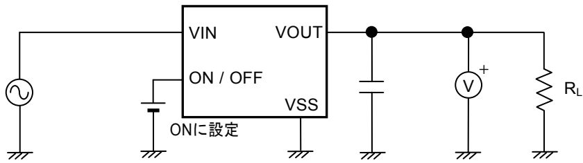
図14 測定回路5
