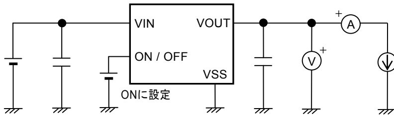
図10 測定回路1
