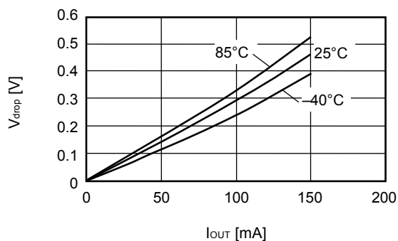
S-1323B30
