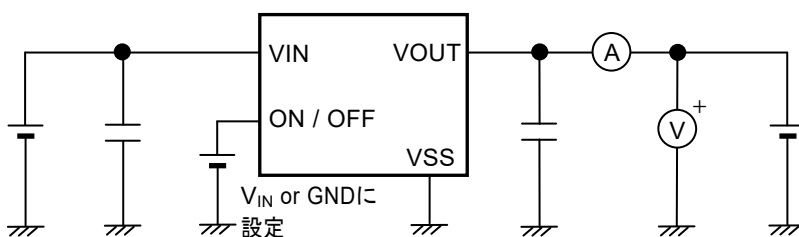
図13 測定回路3
