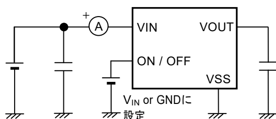
図12 測定回路2
