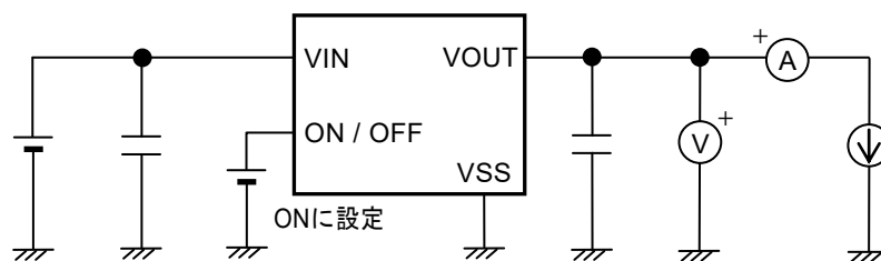
図11 測定回路1
