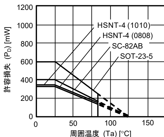
図9 パッケージ許容損失 (基板実装時)
