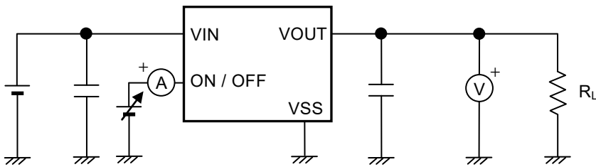
図13 測定回路4
