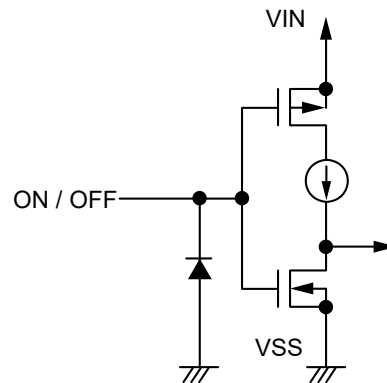
図19 S-1312シリーズB / Dタイプ
