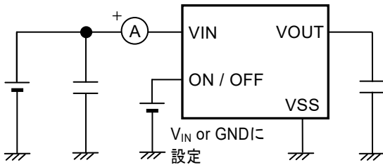
図11 測定回路2
