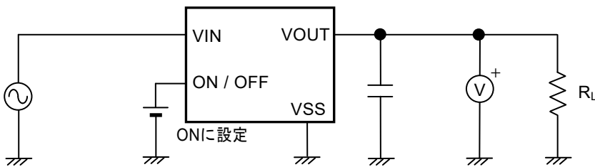
図14 測定回路5
