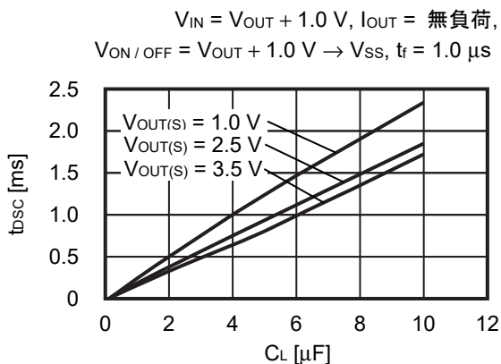
図21 S-1312シリーズA/Bタイプ (放電シャント機能あり)
