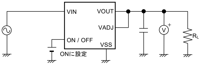
図15 測定回路11
