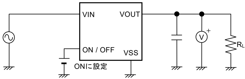
図9 測定回路5
