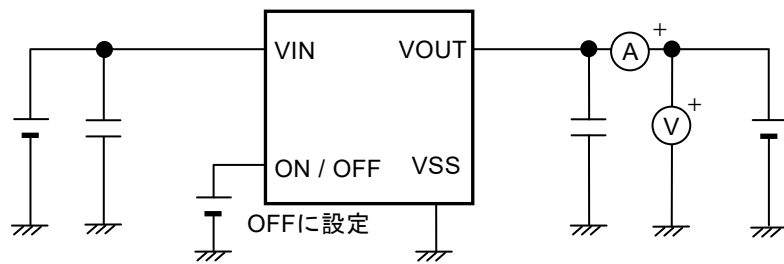
図10 測定回路6
