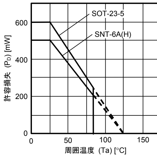
図5 パッケージ許容損失 (基板実装時)
