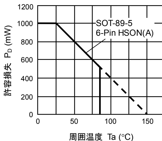
図4 パッケージ許容損失 (基板実装時)
