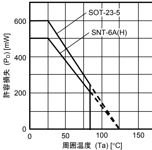
図4 パッケージ許容損失 (基板実装時)
