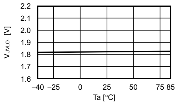
2.16 UVLO検出電圧 ( V_{UVLO-} ) - 温度 ( T_a )
