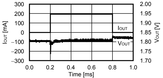
3.4.2 I_{OUT} = 0.1\text{ mA} \rightarrow 200\text{ mA} \rightarrow 0.1\text{ mA}
