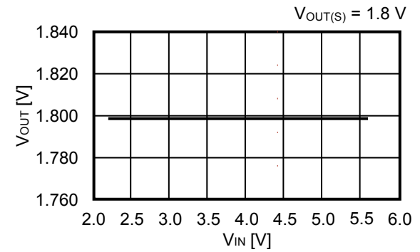
1.4 出力電圧 (V OUT ) – 入力電圧 (V IN )
