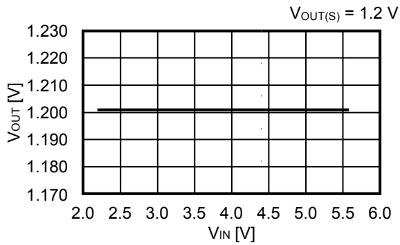
1.3 出力電圧 (V OUT ) – 入力電圧 (V IN )
