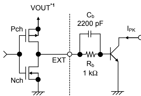
図 20 外付けトランジスタ周辺回路
