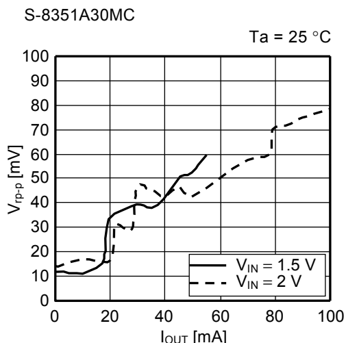
図15 出力電流 ( I_{OUT} ) - リップル電圧 ( V_{ripple} ) 特性 図16 出力電流 ( I_{OUT} ) - リップル電圧 ( V_{ripple} ) 特性
