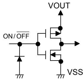
図 17 ON/OFF 端子の構造
