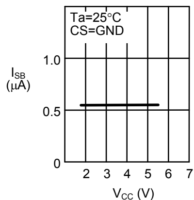
1.12 待機時消費電流 I_{SB} — 電源電圧 V_{CC}
