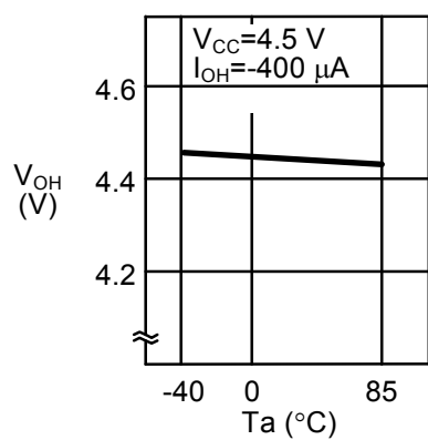
1.17 高レベル出力電圧 V_{OH} — 周囲温度 T_a
