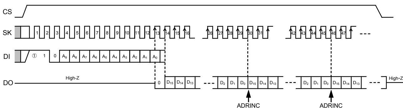
図5 読み出しタイミング
