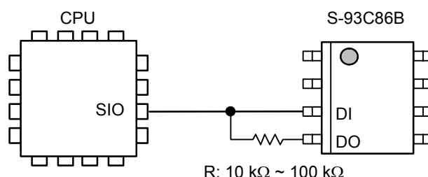
図13 3線式インタフェースの接続法
