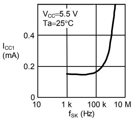
1.6 リード時消費電流 I_{CC1} — クロック周波数 f_{SK}
