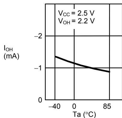
1. 25 高レベル出力電流 I_{OH} —周囲温度 T_a
