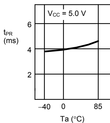
2.3 書き込み時間 t_{PR} —周囲温度 T_a
