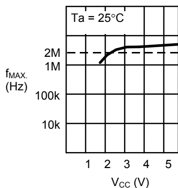
2.1 最大動作周波数 f_{MAX} —電源電圧 V_{CC}
