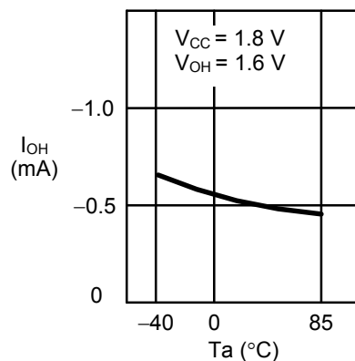
1. 26 高レベル出力電流 I_{OH} —周囲温度 T_a
