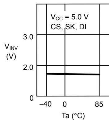
1. 30 入力反転電圧 V_{INV} —周囲温度 T_a
