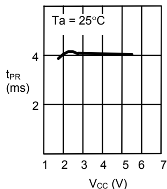
2.2 書き込み時間 t_{PR} —電源電圧 V_{CC}
