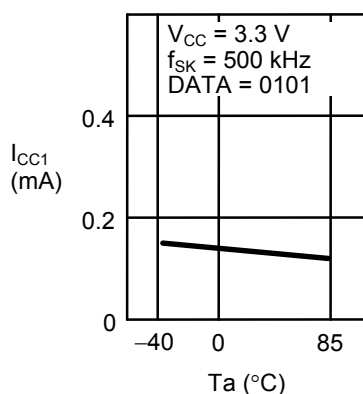
1.2 リード時消費電流 I_{CC1} —周囲温度 T_a
