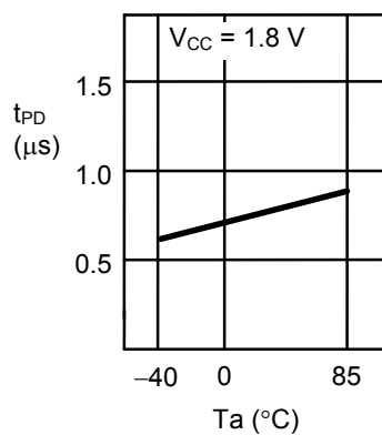
2.8 データ出力遅延時間 t_{PD} —周囲温度 T_a
