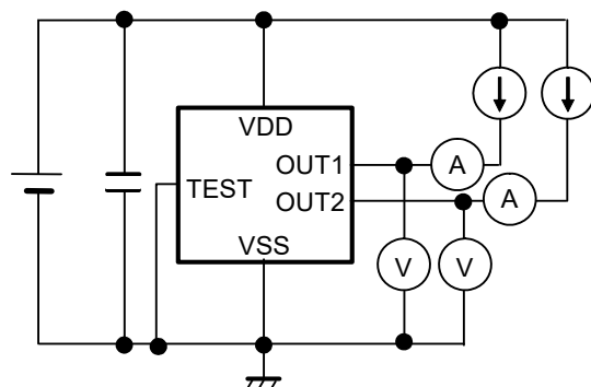
図7 測定回路2
