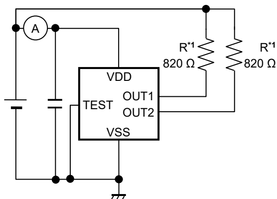
図6 測定回路1
