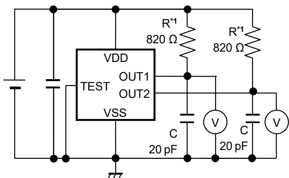
図8 測定回路3
