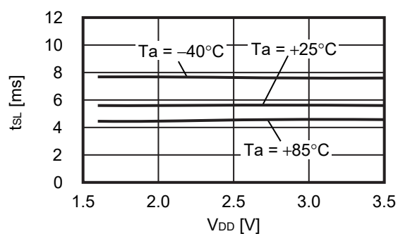
5.8 スリープモード時間 ( t_{SL} ) - 電源電圧 ( V_{DD} )
