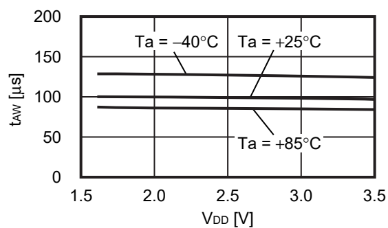
5.6 アウエイクモード時間 ( t_{AW} ) - 電源電圧 ( V_{DD} )
