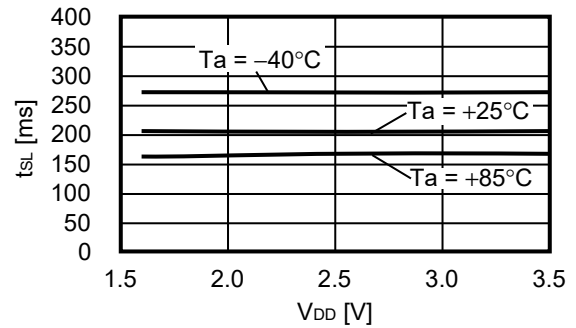
3.8 スリープモード時間 ( t_{SL} ) - 電源電圧 ( V_{DD} )
