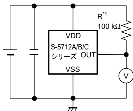
図9 測定回路5
