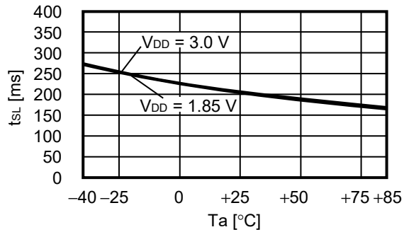
3.7 スリープモード時間 ( t_{SL} ) - 温度 ( T_a )
