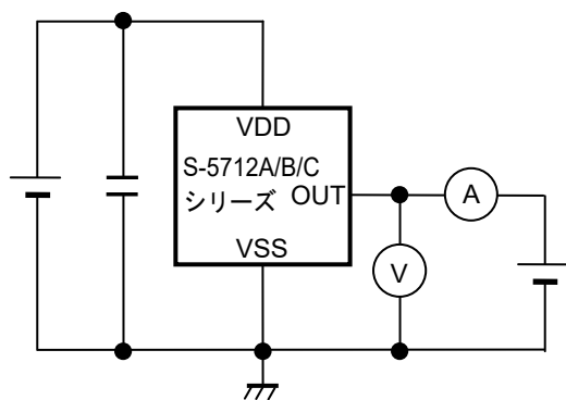
図8 測定回路4
