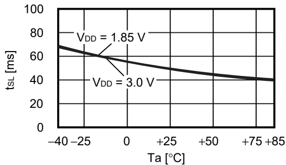
2.7 スリープモード時間 ( t_{SL} ) - 温度 ( T_a )
