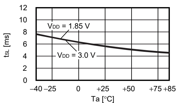
5.7 スリープモード時間 ( t_{SL} ) - 温度 ( T_a )
