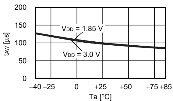
5.5 アウエイクモード時間 ( t_{AW} ) - 温度 ( T_a )
