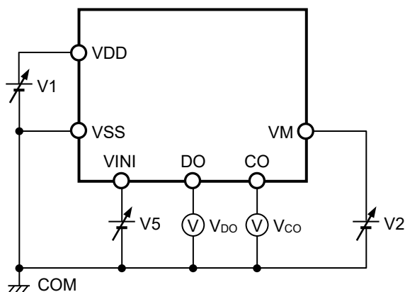
図4 測定回路2
