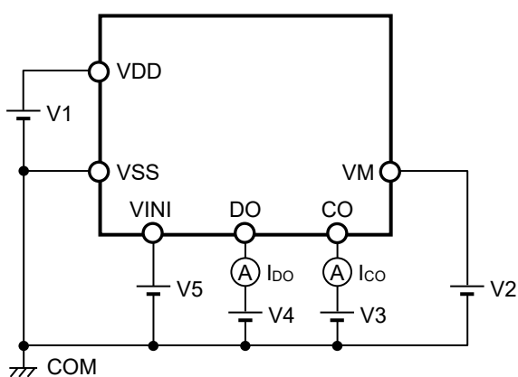
図6 測定回路4
