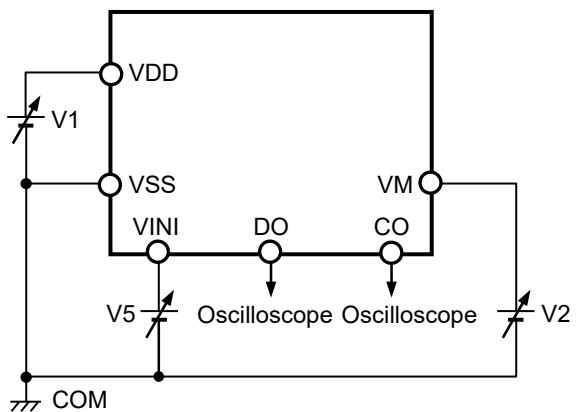
図7 測定回路5
