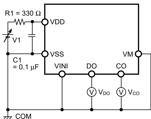
図3 測定回路1
