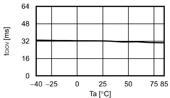
3.10 t_{CIOV} - T_a
