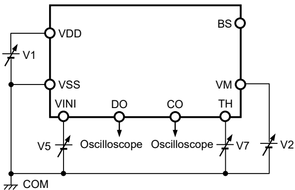
図7 測定回路5
