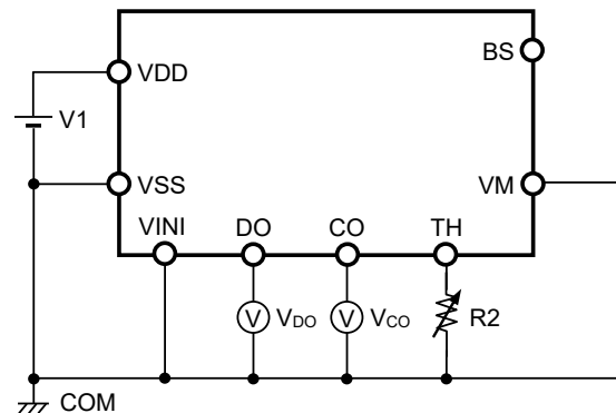
図8 測定回路6
