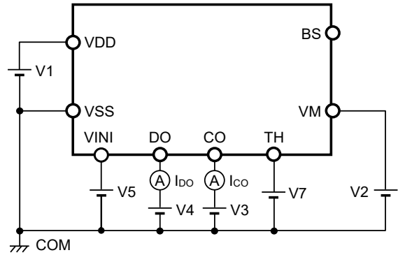
図6 測定回路4
