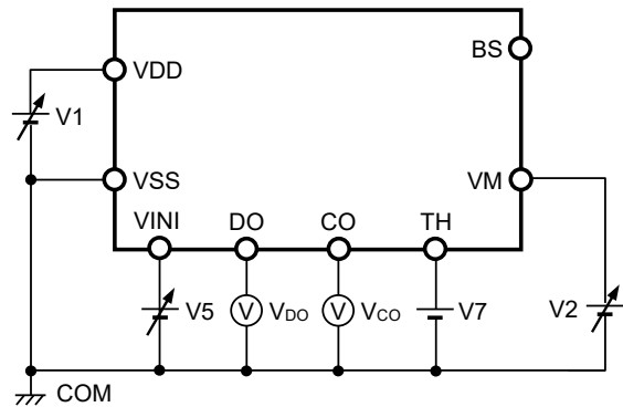
図4 測定回路2
