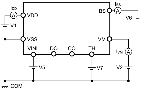
図5 測定回路3
