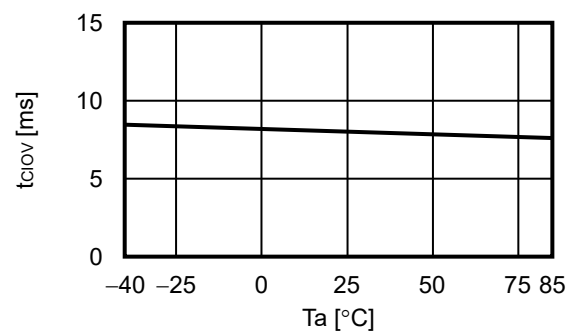
3.8 t_{CIOV} - T_a
