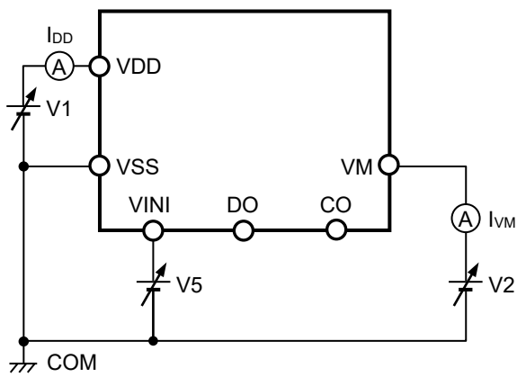
図5 測定回路3
