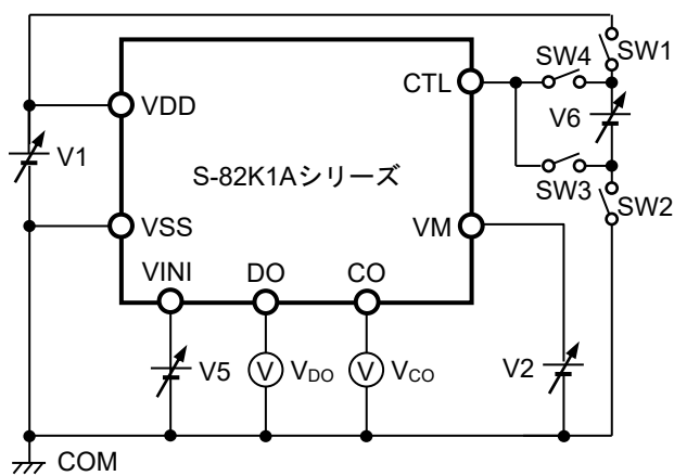
図4 測定回路2
