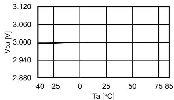
2.4 V_{BU} - T_a
