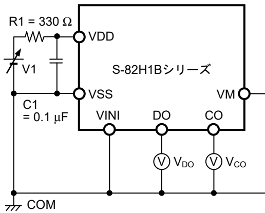
図3 測定回路1
