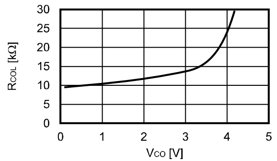
4.2 R_{COL} - V_{CO}
