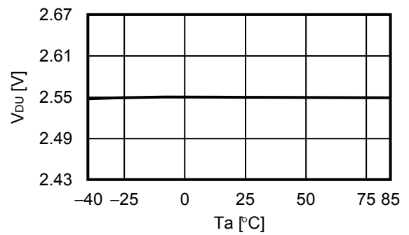
2.4 V_{DU} - T_a
