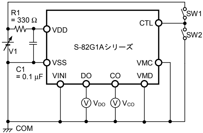
図3 測定回路1
