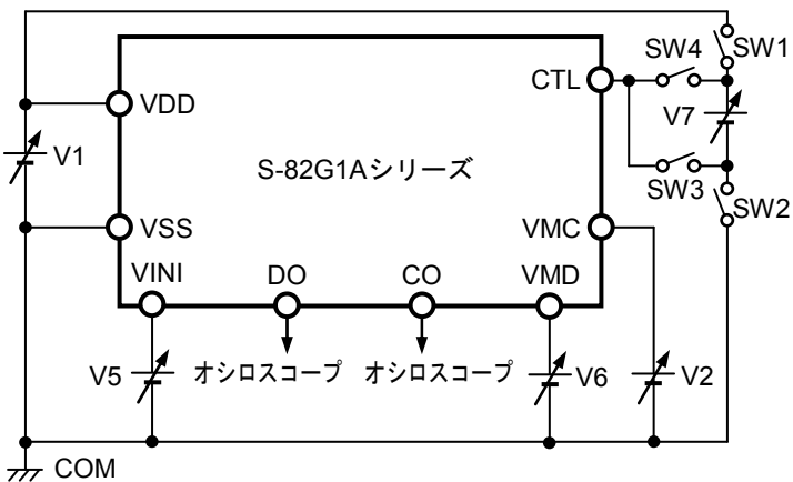
図7 測定回路5
