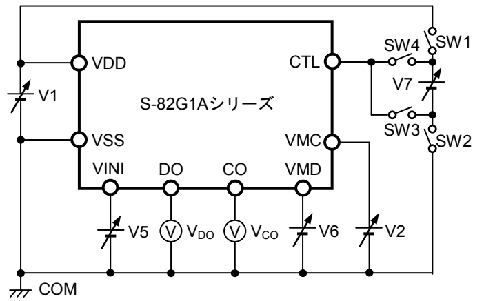
図4 測定回路2
