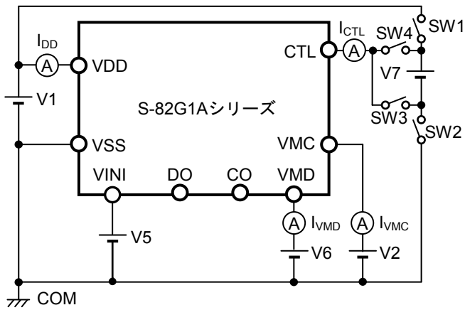
図5 測定回路3
