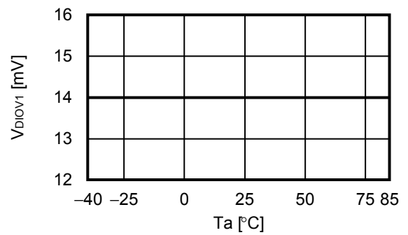
2.6 V_{DIOV1} - T_a
