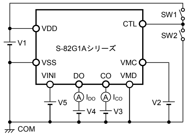
図6 測定回路4
