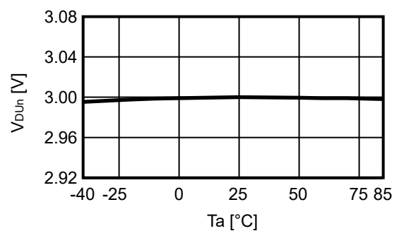
2.4 V_{DUH} - T_a
