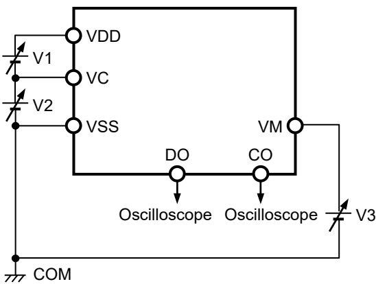
図8 測定回路5
