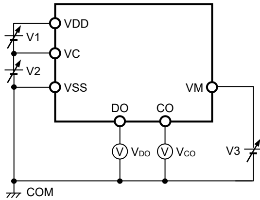
図5 測定回路2
