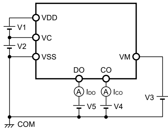
図7 測定回路4
