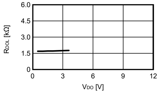
4.4 R_{DOL} - V_{DO}
