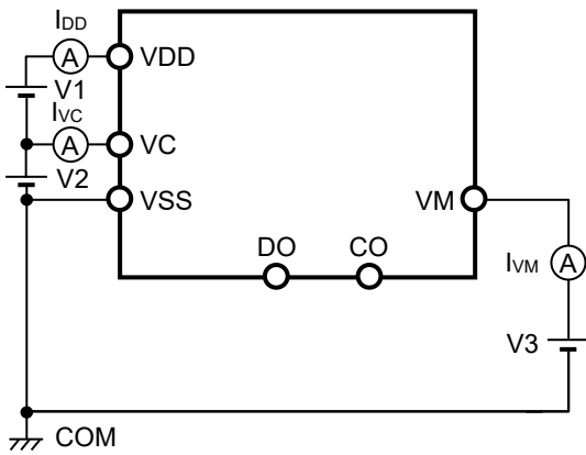
図6 測定回路3
