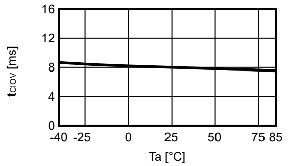
3.10 t_{CIOV} - T_a
