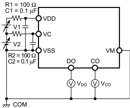
図4 測定回路1
