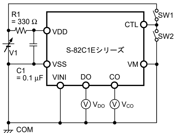
図3 測定回路1
