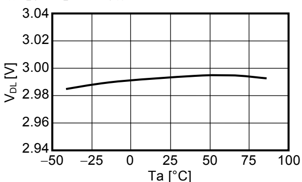
過放電検出電圧-温度特性
