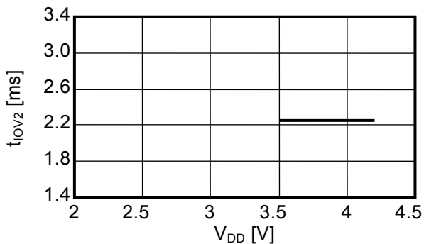
過電流2検出遅延時間－電源電圧特性
