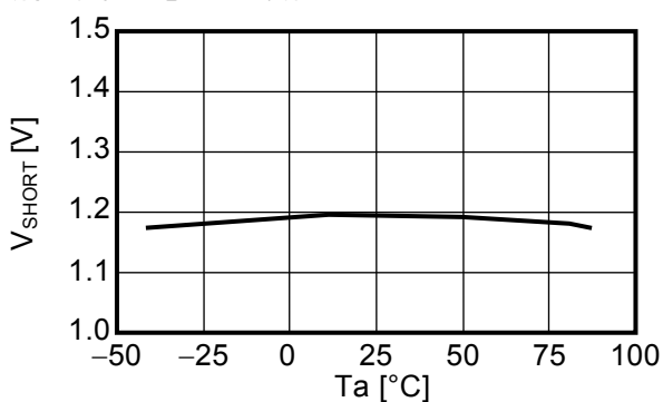
負荷短絡検出電圧-温度特性
