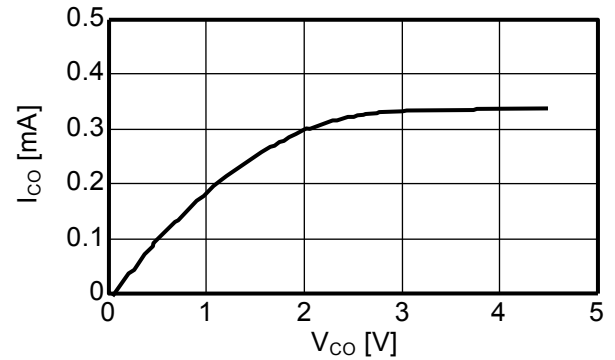
CO端子シンク電流特性 V_{DD} = 4.5\text{ V} , V_M = V_{SS} = 0\text{ V}
