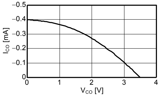
CO端子ソース電流特性 V_{DD} = 3.5\text{ V} , V_M = V_{SS} = 0\text{ V}
