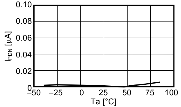
パワーダウン時消費電流－温度特性
