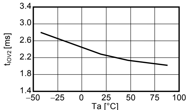
過電流2検出遅延時間－温度特性
