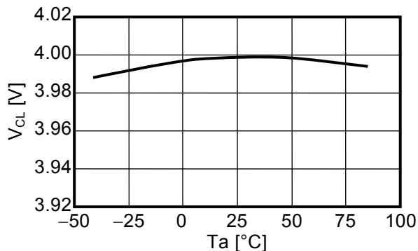
過充電解除電圧-温度特性
