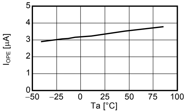
通常動作時消費電流－温度特性
