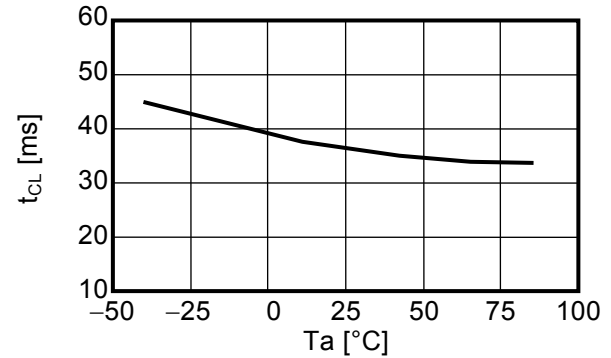
過充電解除遅延時間－温度特性
