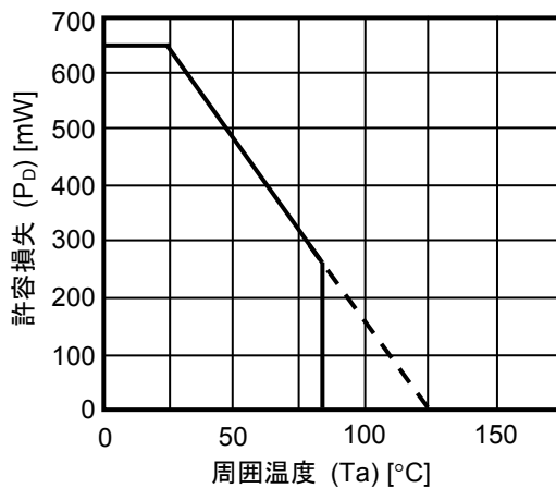
(1) 基板実装時
