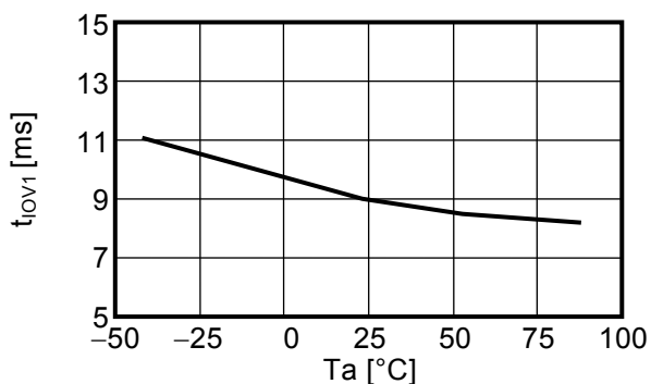
過電流1検出遅延時間－温度特性
