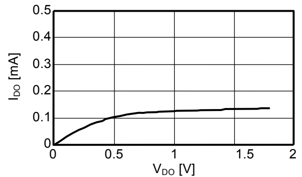
DO端子シンク電流特性 V_{DD} = 1.8\text{ V} , V_M = V_{SS} = 0\text{ V}
