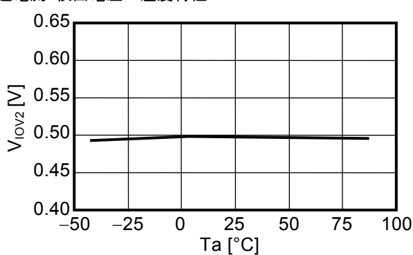
過電流2検出電圧-温度特性
