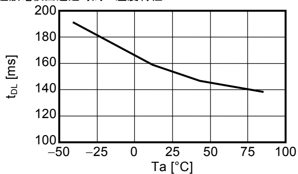
過放電検出遅延時間－温度特性
