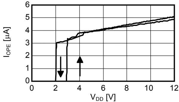
消費電流－電源電圧特性
