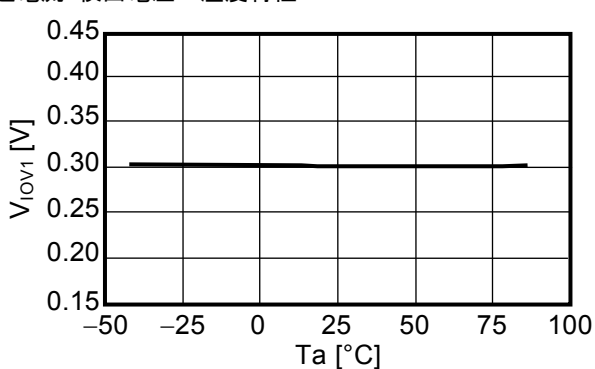
過電流1検出電圧-温度特性
