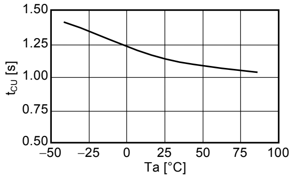
過充電検出遅延時間－温度特性
