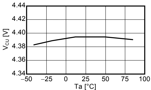
過充電検出電圧-温度特性
