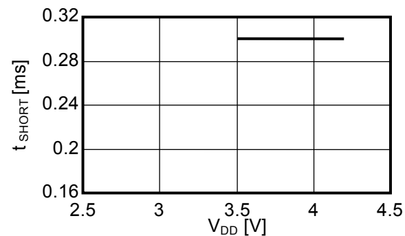
負荷短絡検出遅延時間－電源電圧特性
