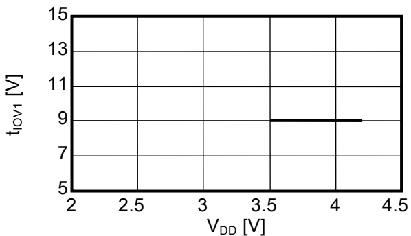
過電流1検出遅延時間－電源電圧特性
