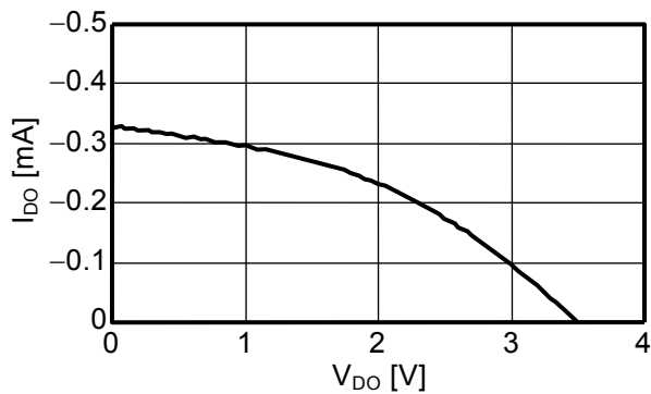
DO端子ソース電流特性 V_{DD} = 3.5\text{ V} , V_M = V_{SS} = 0\text{ V}
