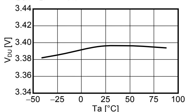
過放電解除電圧-温度特性
