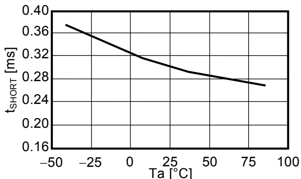
負荷短絡検出遅延時間－温度特性
