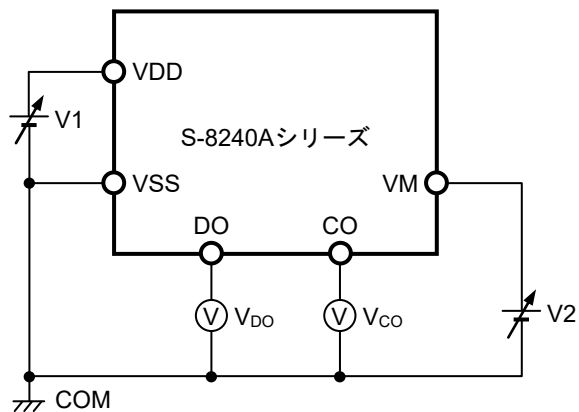
図7 測定回路2
