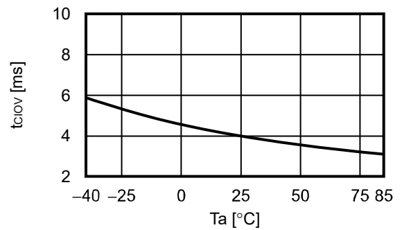
3.8 t_{CIOV} - T_a
