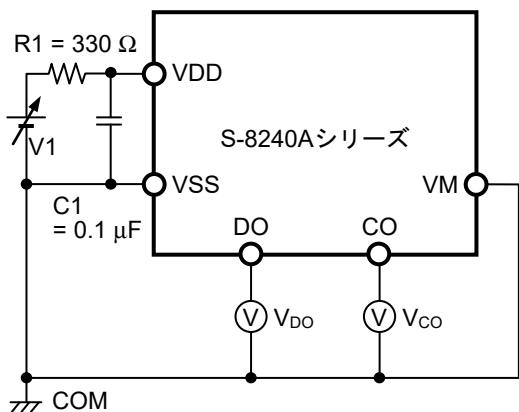
図6 測定回路1
