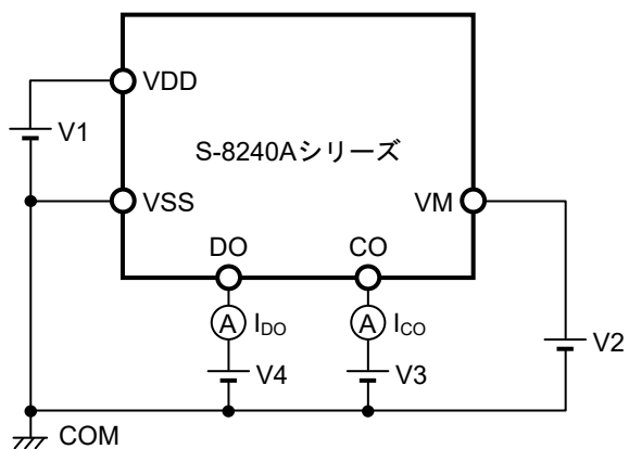
図9 測定回路4
