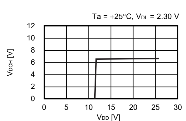
5.2 V_{DO(H)} - V_{DD}
