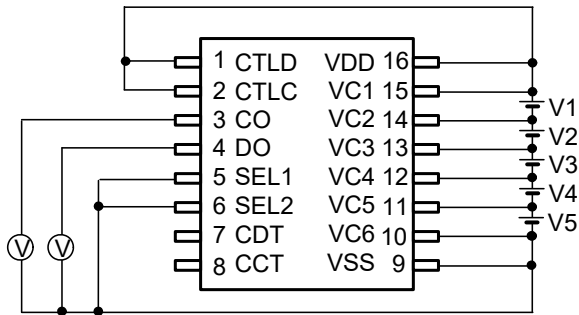
図4 測定回路1
