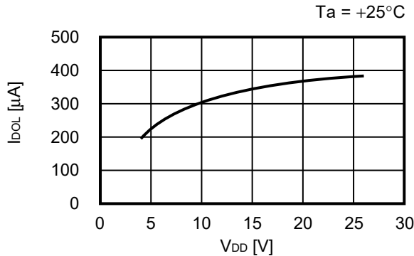
4.3 I_{DO(L)} - V_{DD}
