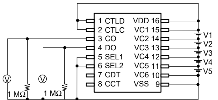
図7 測定回路4
