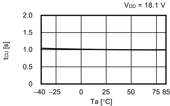
3.1 t_{CU} - T_a
