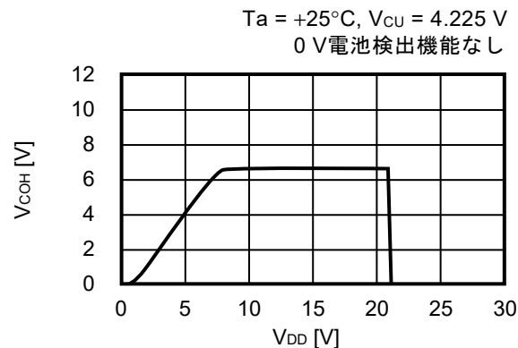
5.1 V_{CO(H)} - V_{DD}
