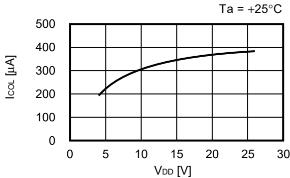
4.1 I_{CO(L)} - V_{DD}
