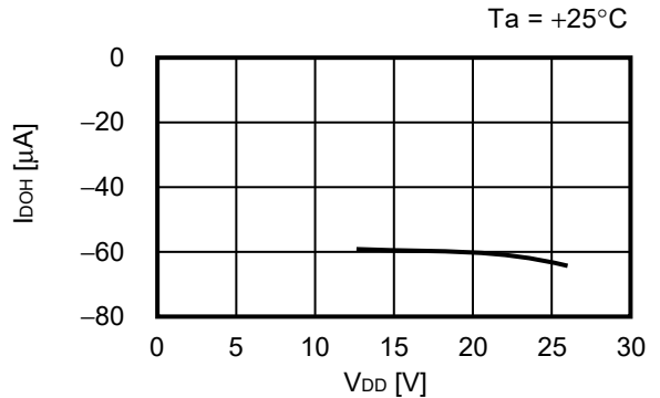
4.4 I_{DO(H)} - V_{DD}
