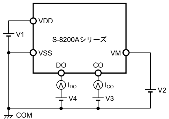
図8 測定回路4
