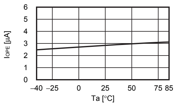
1.1 I_{OPE} - T_a
