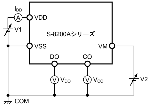
図6 測定回路2
