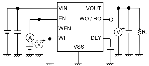
図12 測定回路4
