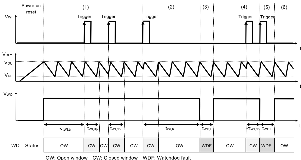
図24 ウォッチドッグタイマ部のタイミングチャート
