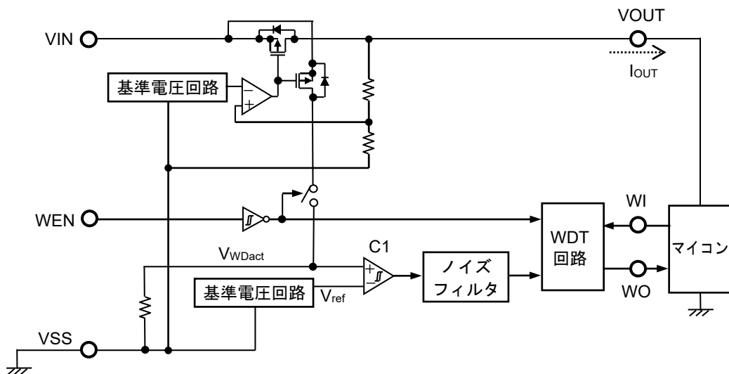
図27 出力電流検出回路の動作説明図
