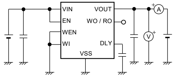
図10 測定回路2
