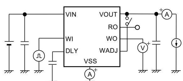
図29 測定回路10
