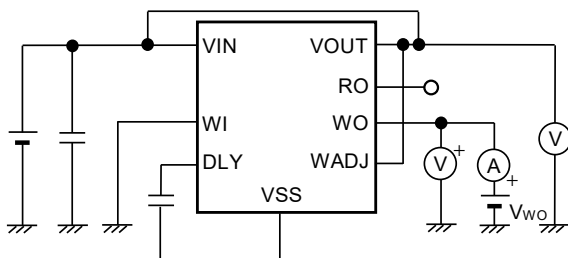
図28 測定回路9
