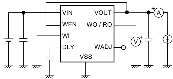
図15 測定回路6
