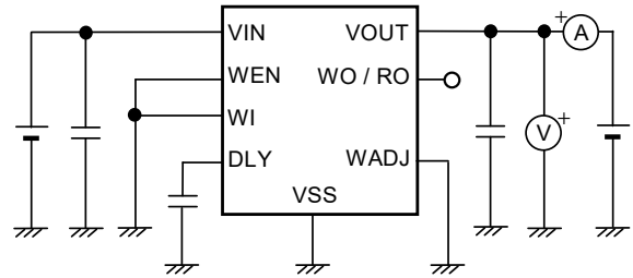
図11 測定回路2
