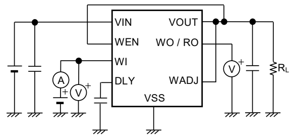
図17 測定回路8
