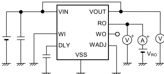
図24 測定回路5
