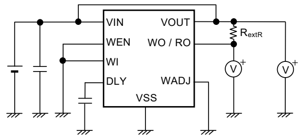
図13 測定回路4
