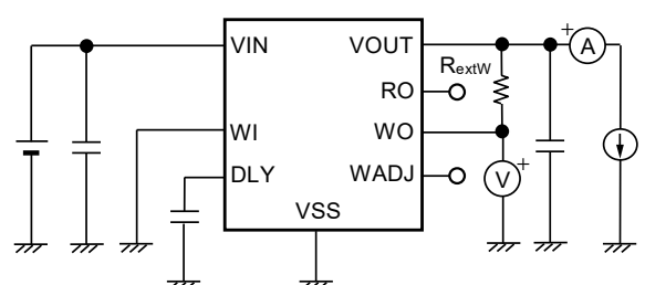
図25 測定回路6
