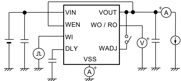
図19 測定回路10
