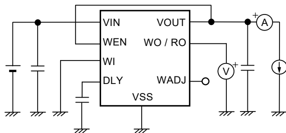
図15 測定回路6
