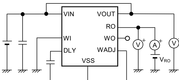
図24 測定回路5
