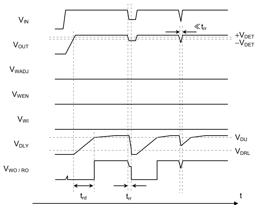
図42 ディテクタ動作例
