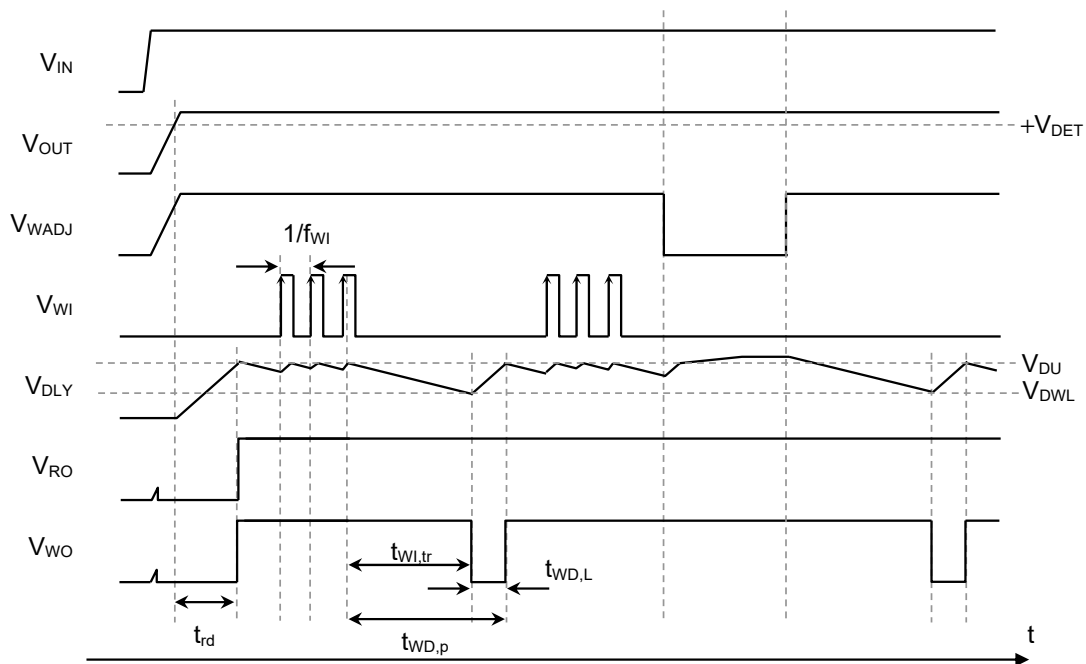
図43 ウォッチドッグタイマ監視動作例
