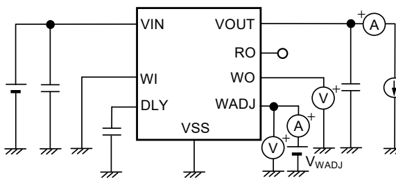
図26 測定回路7
