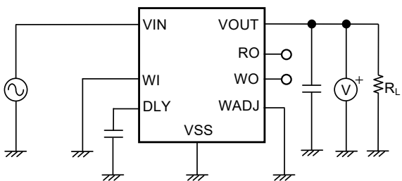
図22 測定回路3
