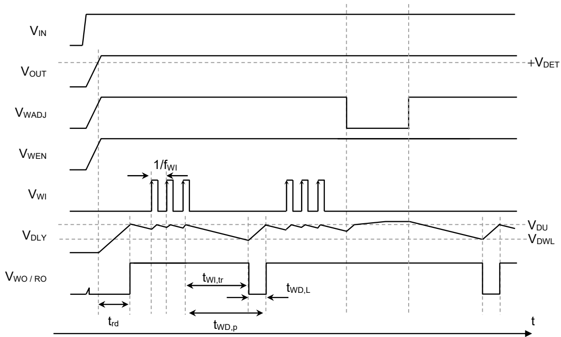
図40 ウォッチドッグタイマ監視動作例1
