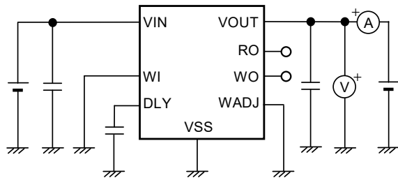
図21 測定回路2
