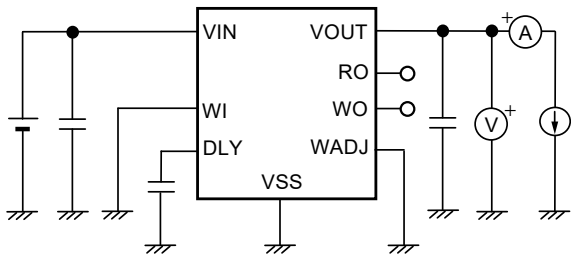
図20 測定回路1
