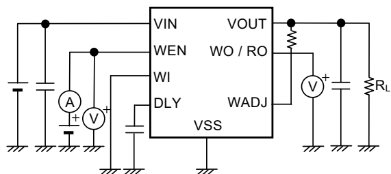
図17 測定回路8
