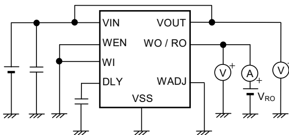
図14 測定回路5
