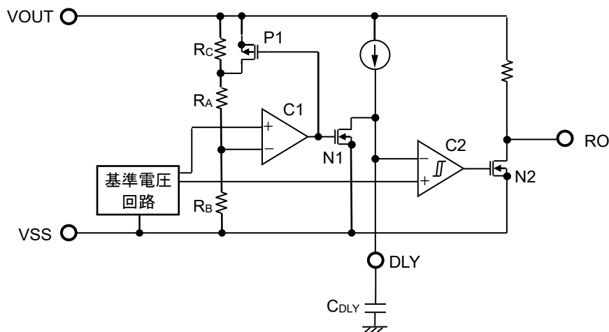
図34 ディテクタ部の動作説明図
