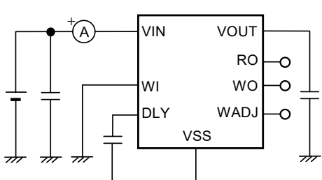
図28 測定回路9
