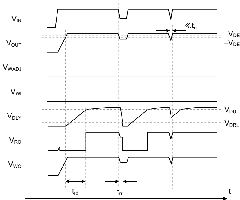
図44 ディテクタ動作例
