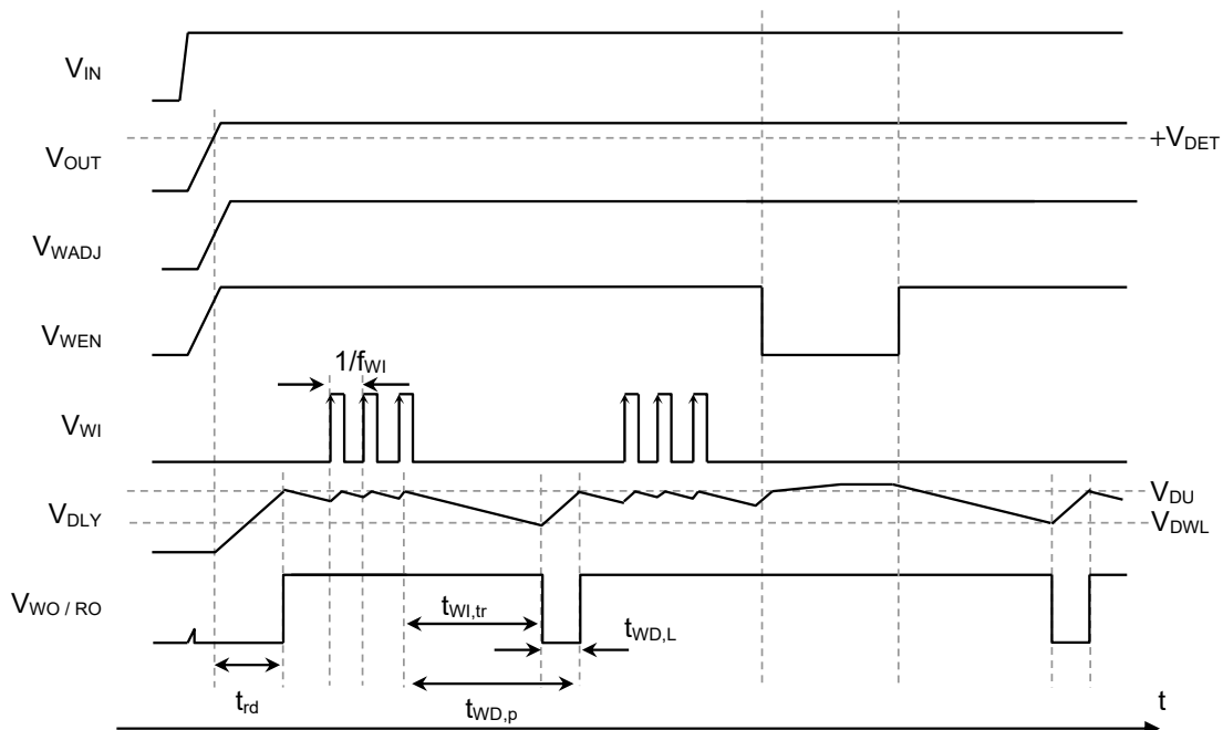
図41 ウォッチドッグタイマ監視動作例2
