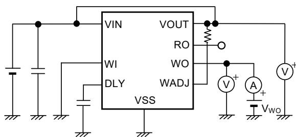
図30 測定回路11
