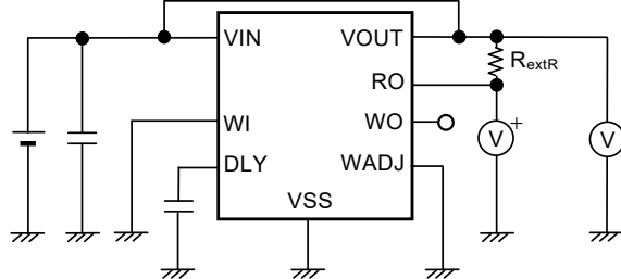
図23 測定回路4
