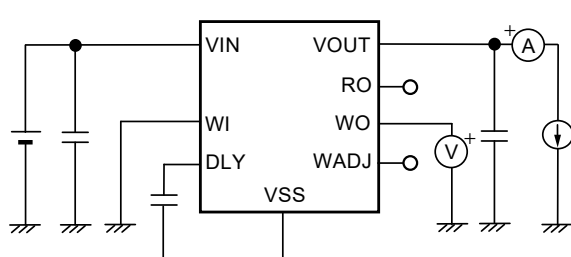
図25 測定回路6
