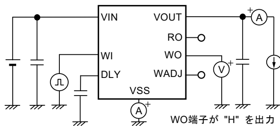
図27 測定回路8
