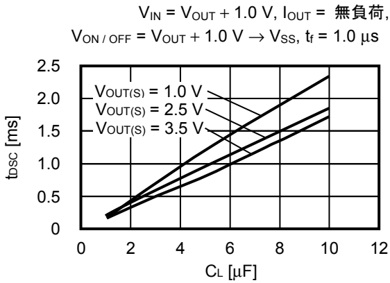
図18 S-19251シリーズA/Bタイプ (放電シャント機能あり)
