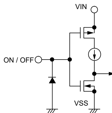
図16 S-19251シリーズB / D タイプ
