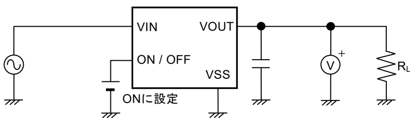
図12 測定回路5
