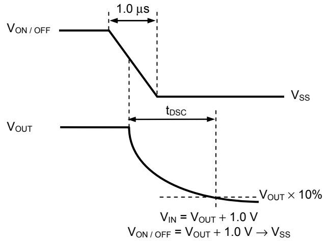
図19 放電時間の測定条件
