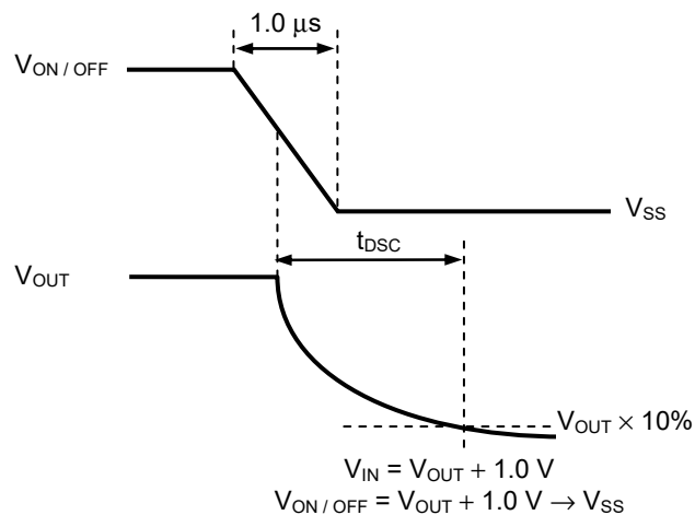
図19 放電時間の測定条件
