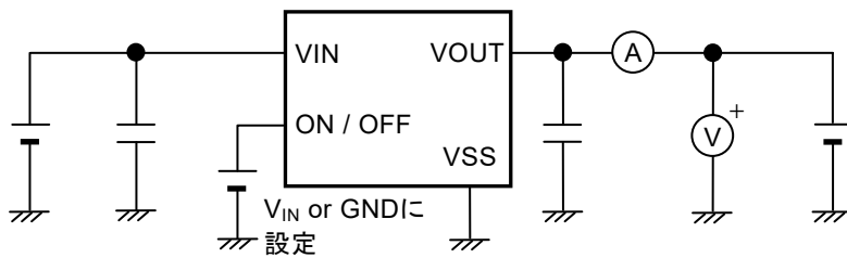
図10 測定回路3
