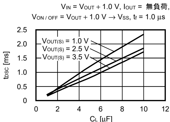
図18 S-19251シリーズA/Bタイプ (放電シャント機能あり)
