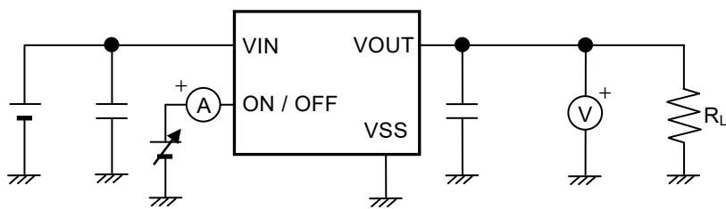
図11 測定回路4
