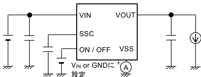
図4 測定回路2
