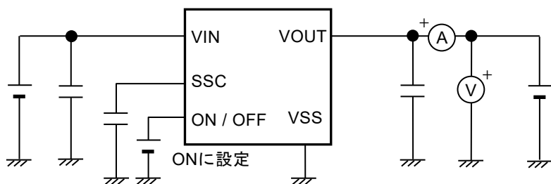
図5 測定回路3
