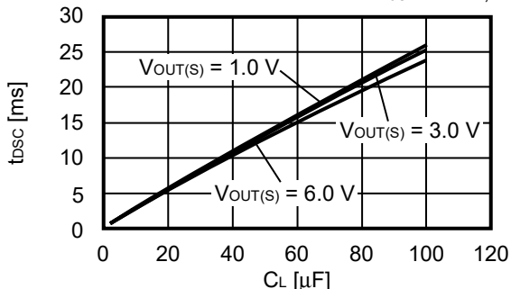
図15 S-19246xxxHシリーズE/Fタイプ (放電シャント機能あり)
