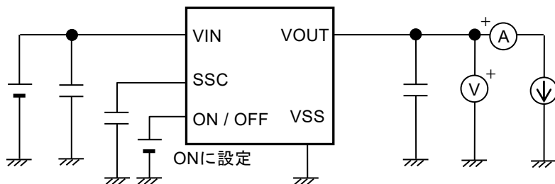
図3 測定回路1
