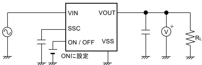
図7 測定回路5
