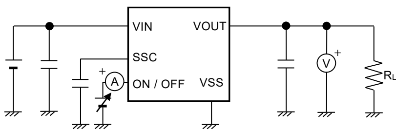
図6 測定回路4
