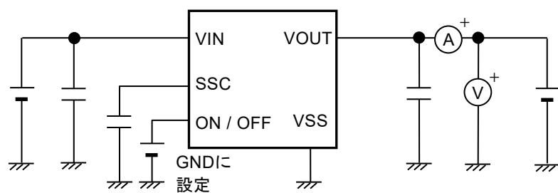
図8 測定回路6
