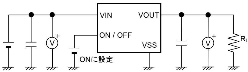
図14 ロードダンプ特性の測定回路
