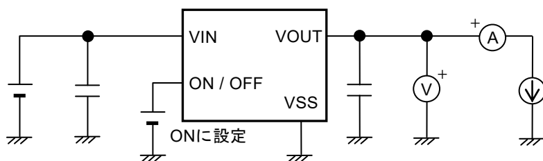
図4 測定回路1
