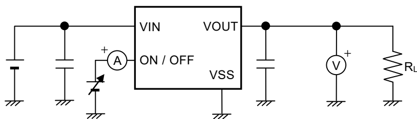
図7 測定回路4
