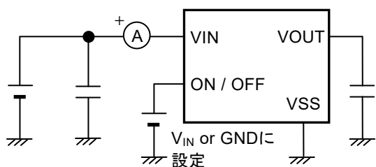
図5 測定回路2
