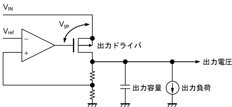
図12 回路図
