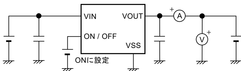
図6 測定回路3
