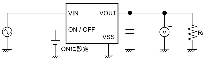
図8 測定回路5
