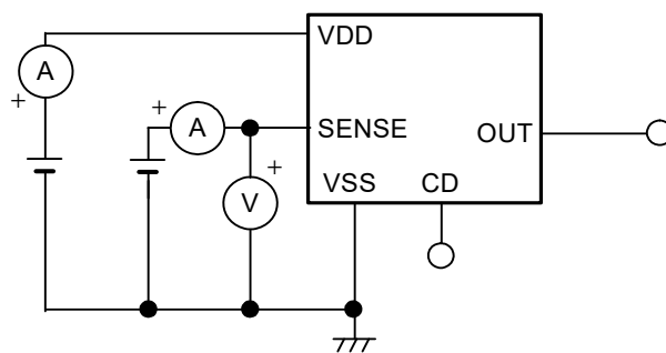
図9 測定回路4
