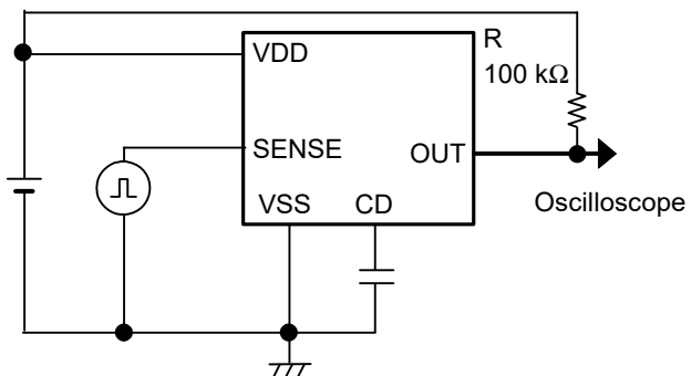
図8 測定回路3
