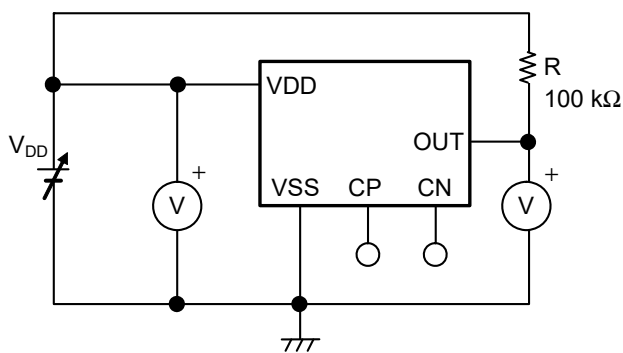
図22 検出電圧、解除電圧の測定回路 (VDD検出品)
