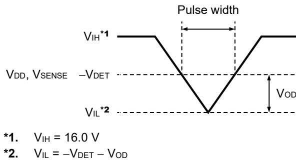
図47 VDD端子、SENSE端子入力電圧波形
