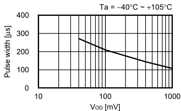
図49 SENSE検出品
