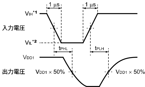
図57 応答時間の測定条件
