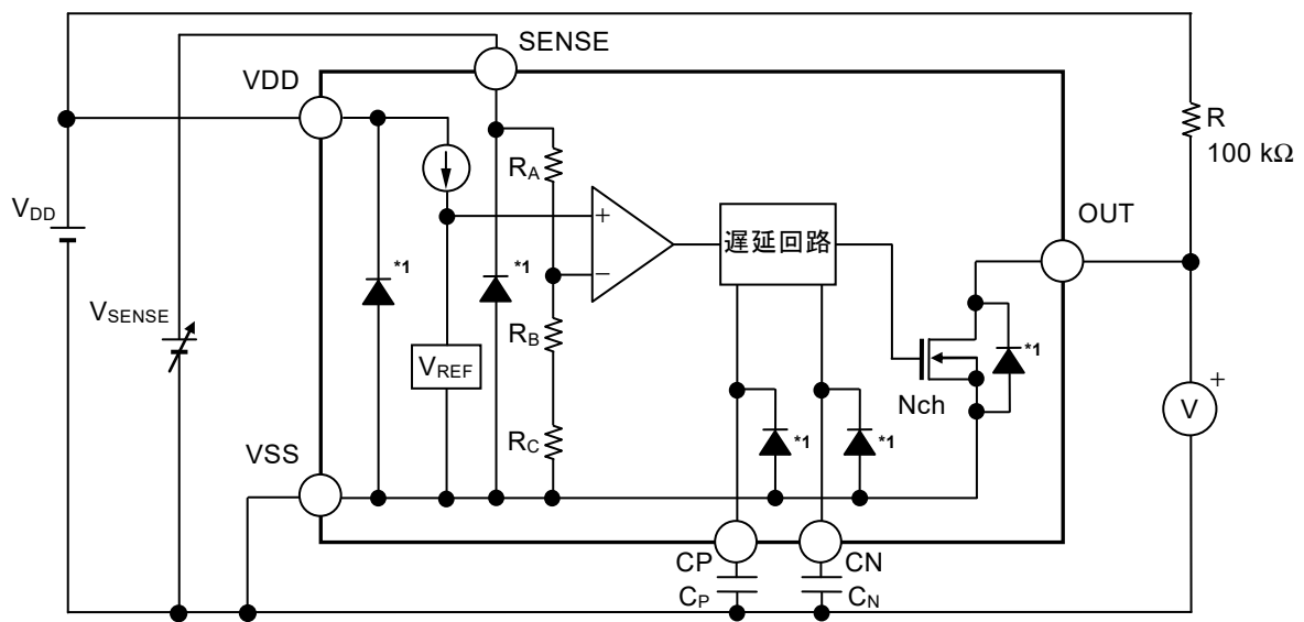
図36 S-19110シリーズQタイプの動作説明図
