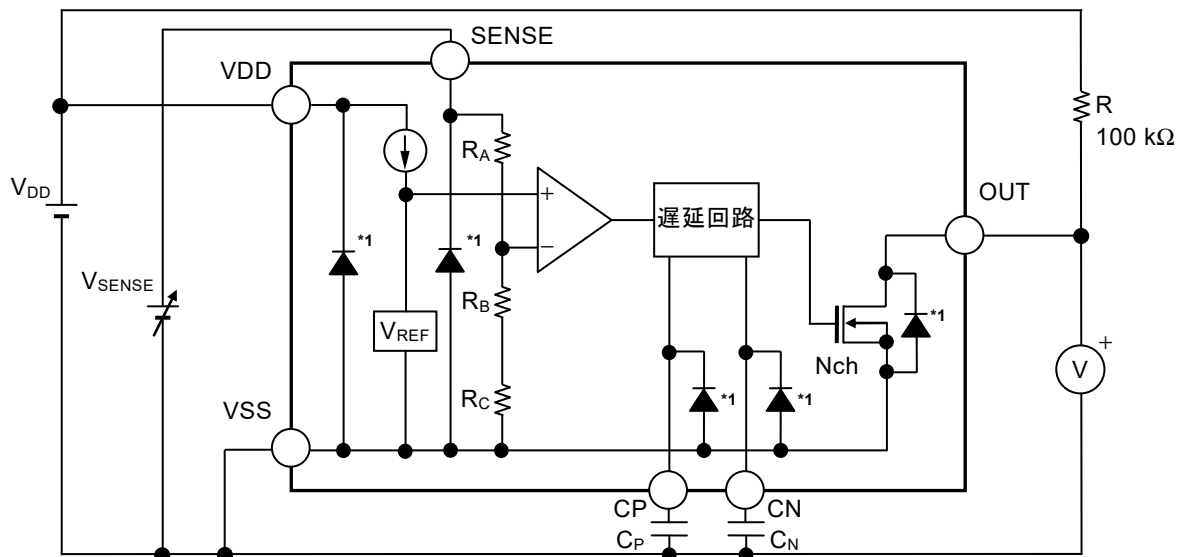
図38 S-19110シリーズRタイプの動作説明図
