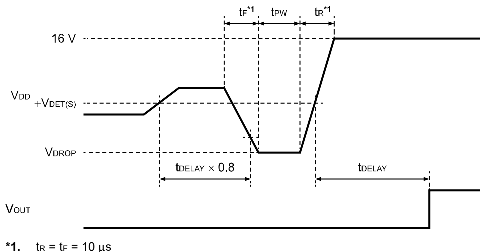
図56 V DD 端子入力電圧波形
