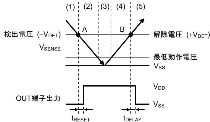
図38 S-19110シリーズRタイプの動作説明図
