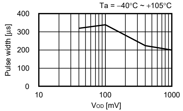
図46 SENSE検出品
