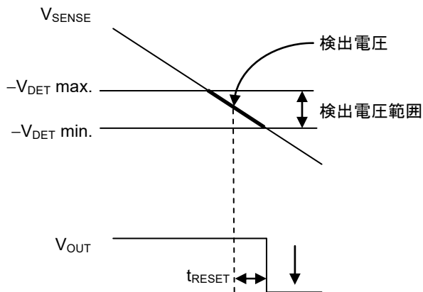
図20 検出電圧 (SENSE検出品)
