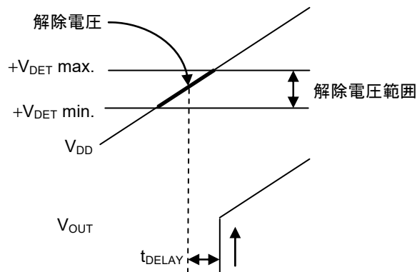
図19 解除電圧 (VDD検出品)
