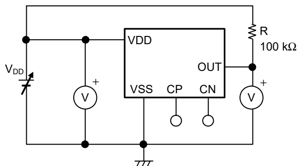
図67 ロードダンプ特性の測定回路
