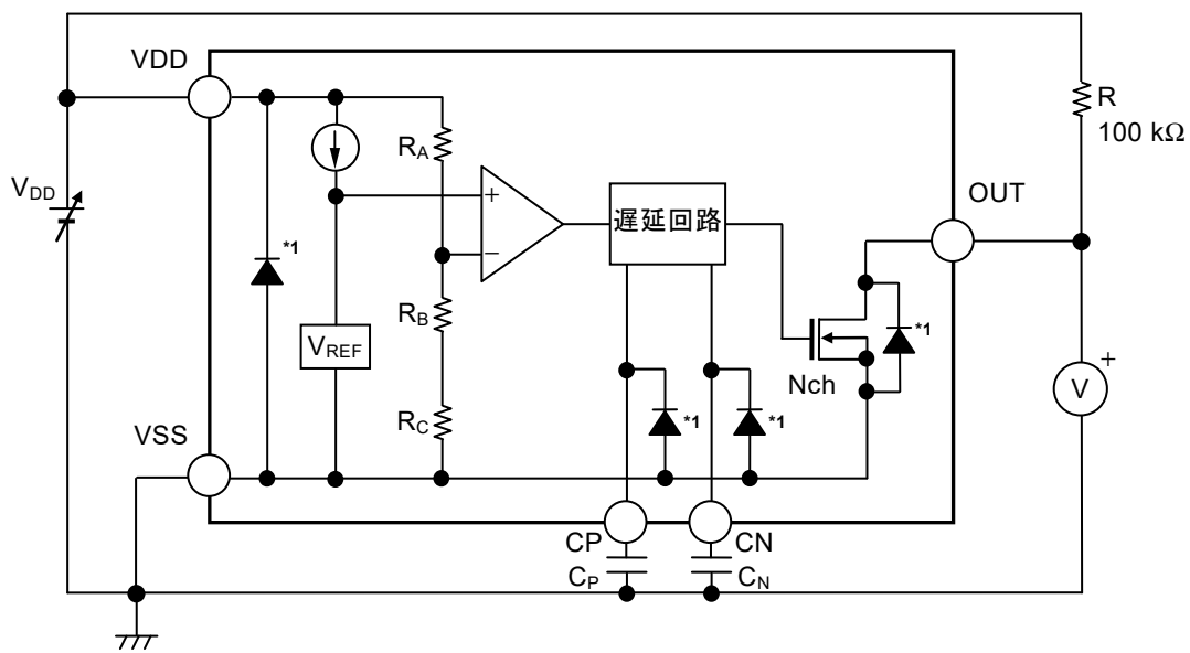
図28 S-19110シリーズLタイプの動作説明図
