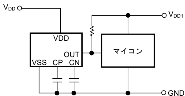
図68 リセット回路例 (VDD検出品)
