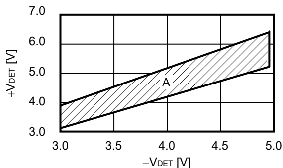
図5 検出電圧、解除電圧設定可能領域
