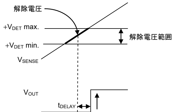
図21 解除電圧 (SENSE検出品)
