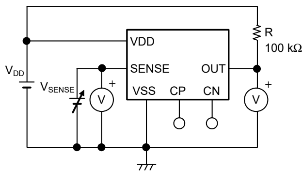
図23 検出電圧、解除電圧の測定回路 (SENSE検出品)
