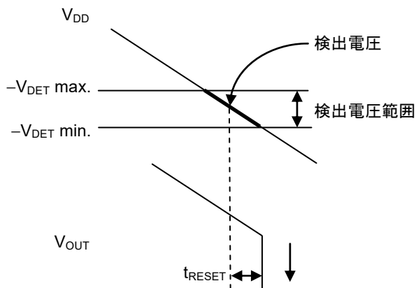
図18 検出電圧 (VDD検出品)
