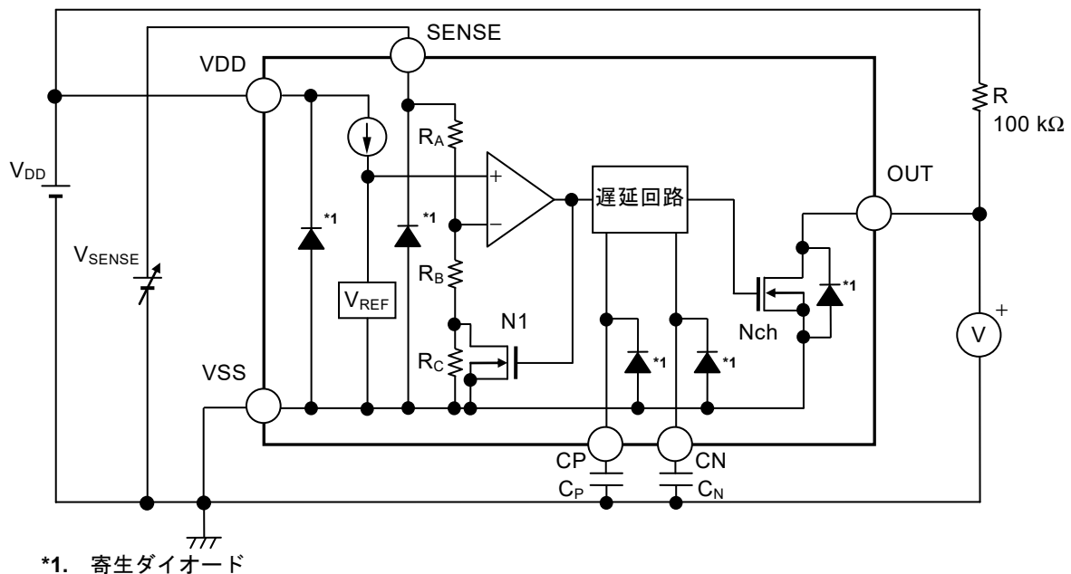
図34 S-19110シリーズPタイプの動作説明図
