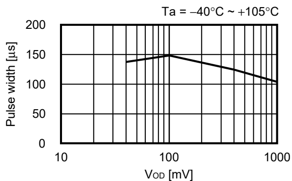
図48 VDD検出品
