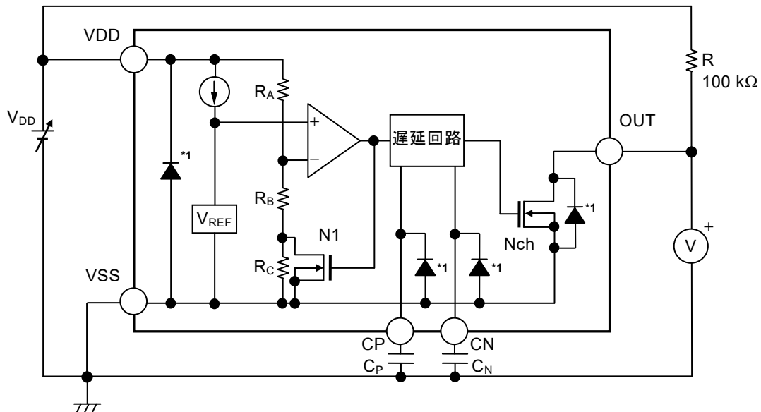
図26 S-19110シリーズKタイプの動作説明図
