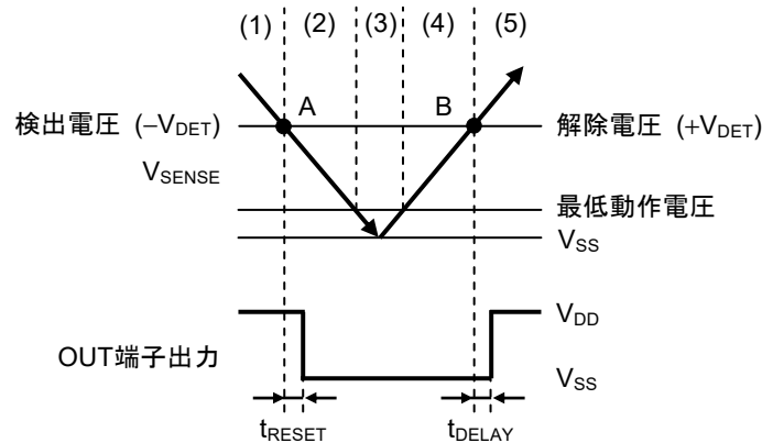
図36 S-19110シリーズQタイプの動作説明図
