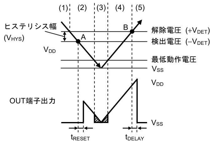
図26 S-19110シリーズKタイプの動作説明図
