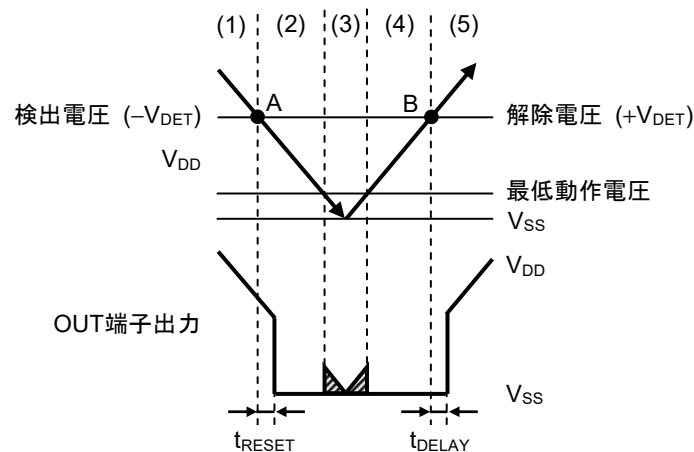
図28 S-19110シリーズLタイプの動作説明図
