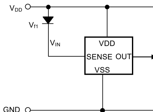
図37 ダイオードを用いた検出電圧の変更 (CMOS出力品)
