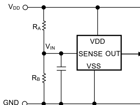
図35 分割抵抗を用いた検出電圧の変更 (CMOS出力品)
