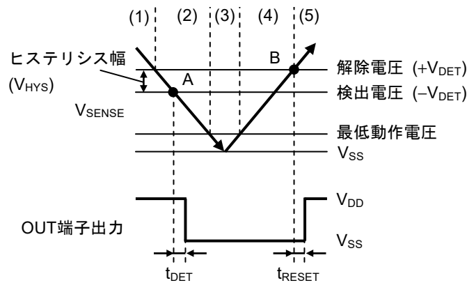
図22 S-19102/19108シリーズCタイプのタイミングチャート
