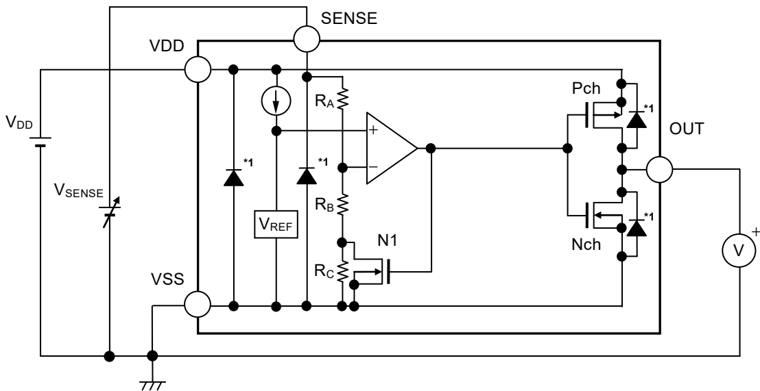
図21 S-19102/19108シリーズCタイプの動作説明図
