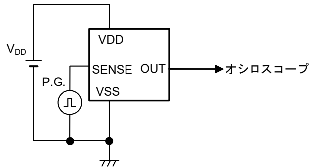
図10 測定回路4 (CMOS出力品)
