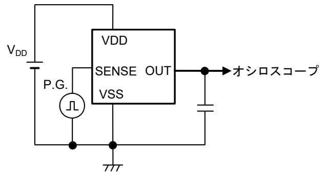
図31 応答時間の測定回路 (CMOS出力品)
