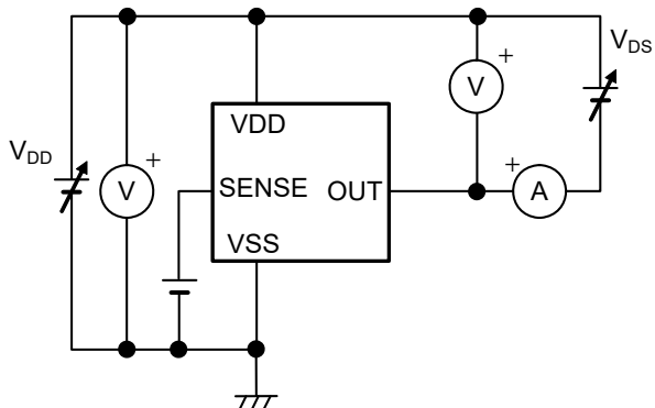
図11 測定回路5
