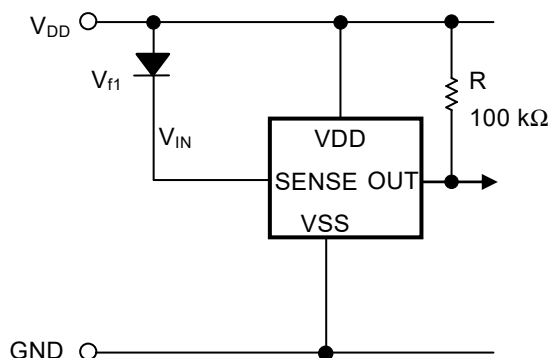
図36 ダイオードを用いた検出電圧の変更 (Nchオープンドレイン出力品)
