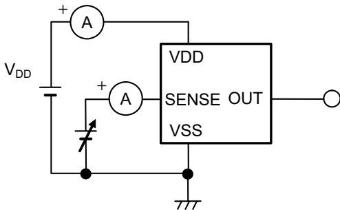
図7 測定回路2
