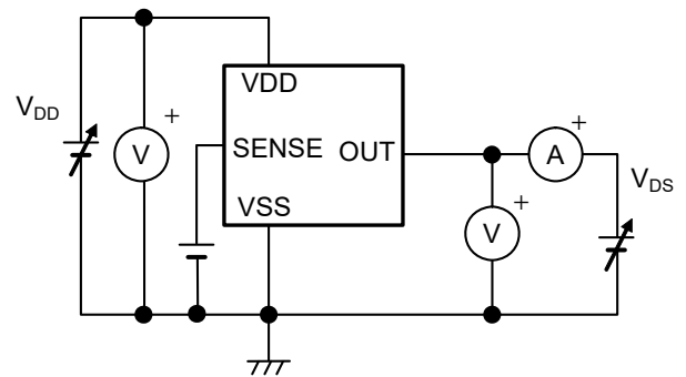
図8 測定回路3
