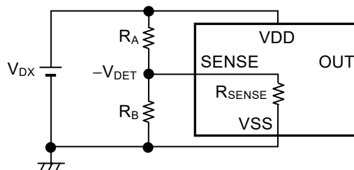
図23 検出電圧外部設定回路
