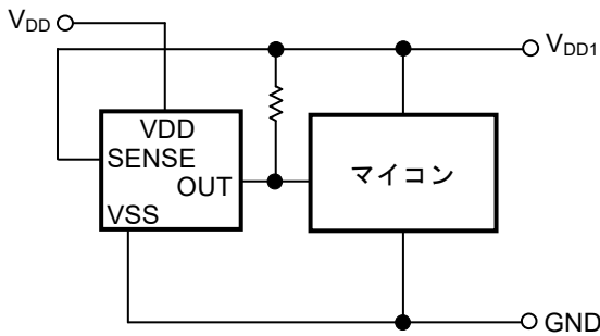
図32 リセット回路例 (Nchオープンドレイン出力品)
