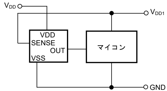
図33 リセット回路例 (CMOS出力品)
