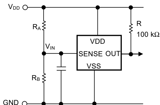
図34 分割抵抗を用いた検出電圧の変更 (Nchオープンドレイン出力品)
