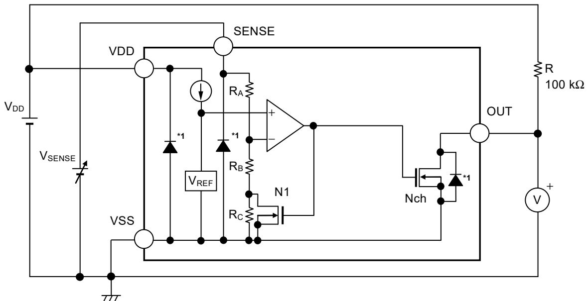
図19 S-19102/19108シリーズNタイプの動作説明図
