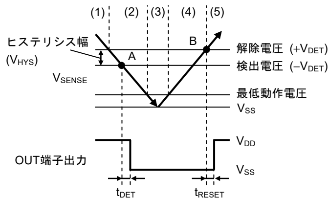
図20 S-19102/19108シリーズNタイプのタイミングチャート
