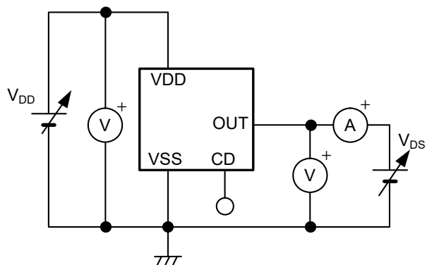
図8 測定回路3
