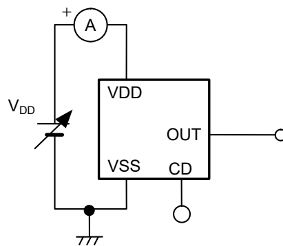
図7 測定回路2
