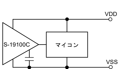
図26 リセット回路例 (CMOS出力品)
