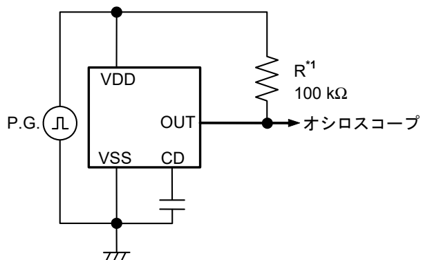
図9 測定回路4
