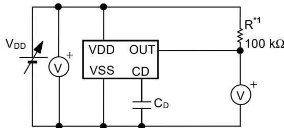
図19 検出電圧、解除電圧の測定回路
