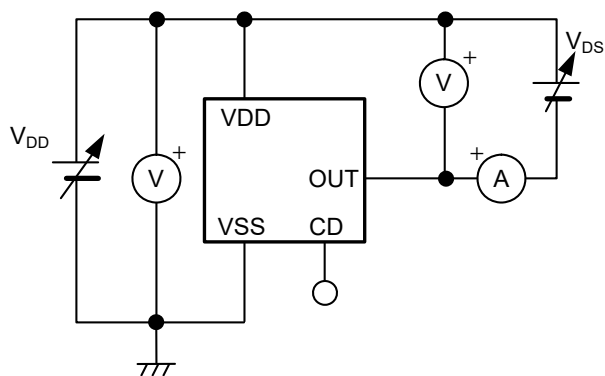
図10 測定回路5
