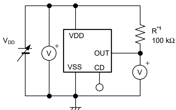
図6 測定回路1
