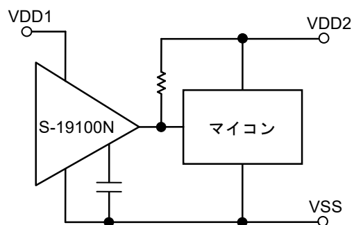
図27 リセット回路例 (Nchオープンドレイン出力品)
