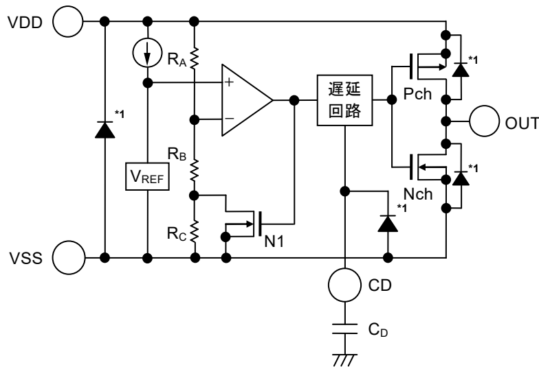
*1. 寄生ダイオード
