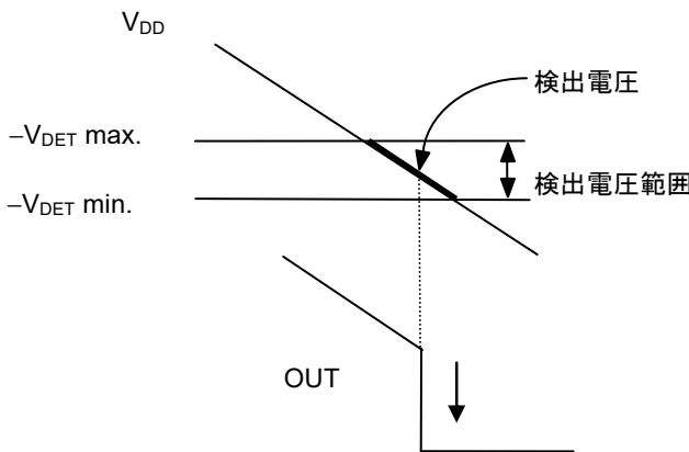
図17 検出電圧
