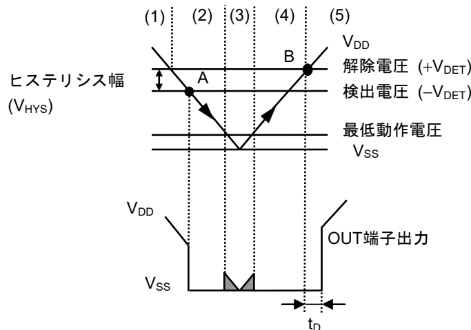
図14 動作説明図2
