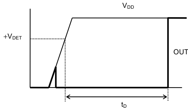
図20 遅延時間
