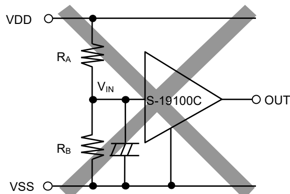
図21 検出電圧変更回路不良事例
