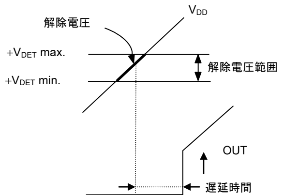
図18 解除電圧
