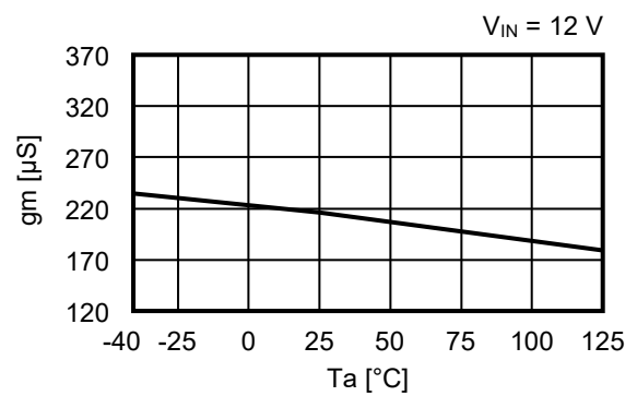
2.14 誤差増幅回路トランスコンダクタンス ( g_m ) – 温度 ( T_a )
