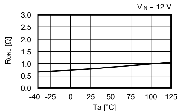
2.10 GATE端子オン抵抗 ( R_{ONL} ) – 温度 ( T_a )
