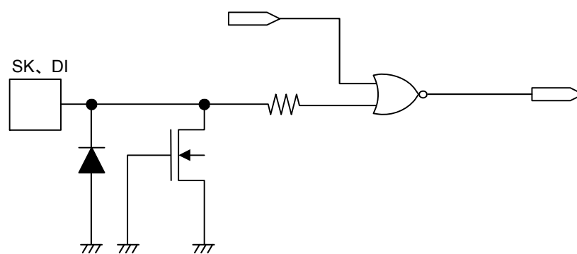
図15 SK, DI端子
