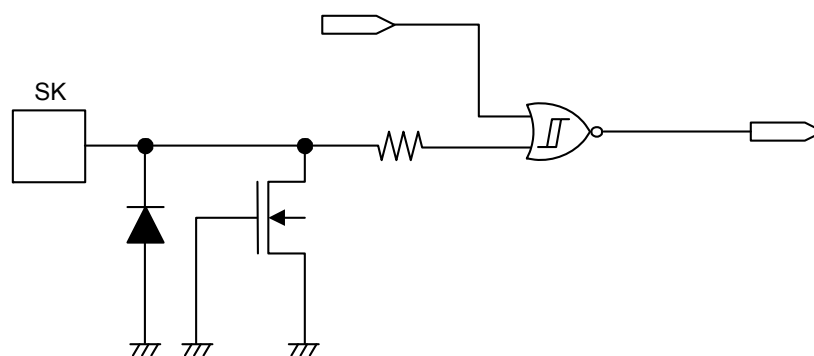
図 22 SK 端子
