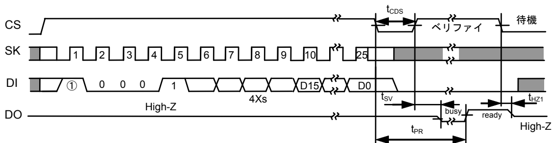
図12 チップ書き込みタイミング (S-93A46A)
