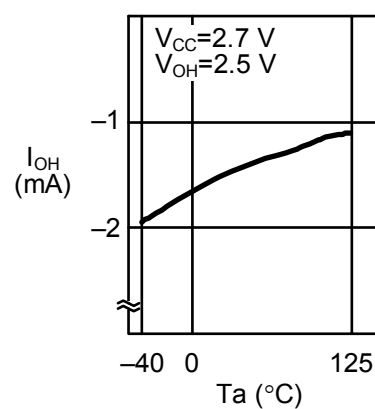
1. 24 高レベル出力電流 I_{OH} —周囲温度 T_a
