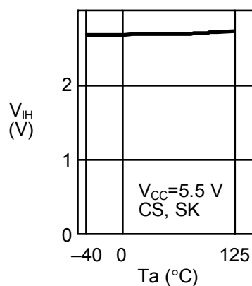
1. 28 高レベル入力電圧 V_{IH} —周囲温度 T_a
