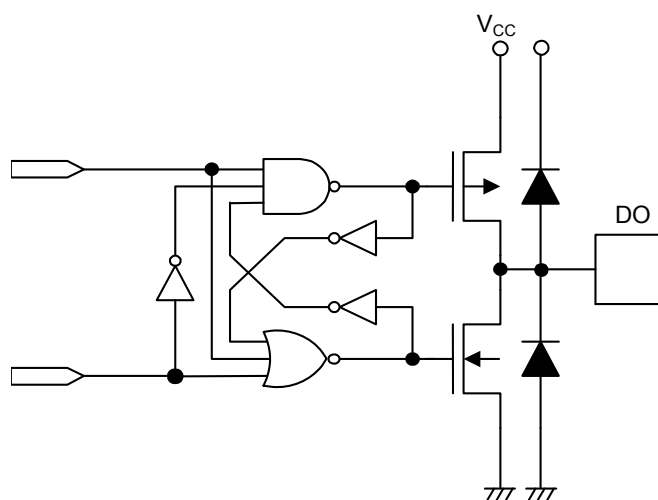
図 25 DO 端子
