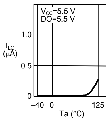
1. 16 出力リーク電流 I_{LO} —周囲温度 T_a
