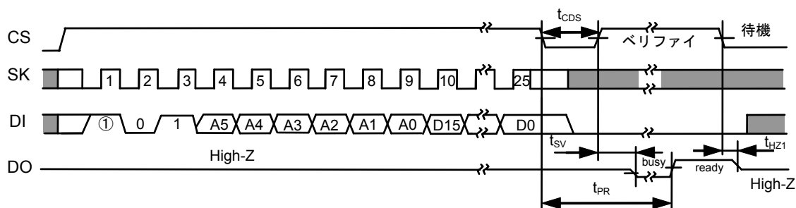
図8 データ書き込みタイミング (S-93A46A)
