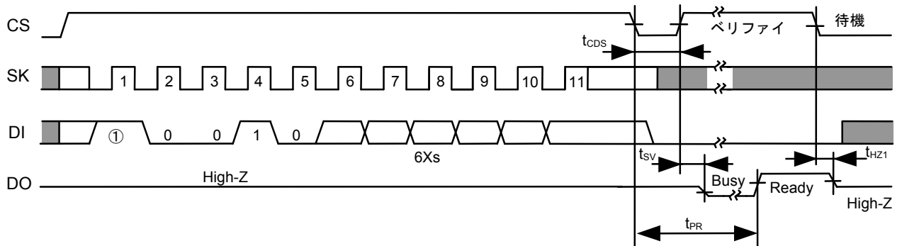
図15 チップ消去タイミング (S-93A56A, S-93A66A)
