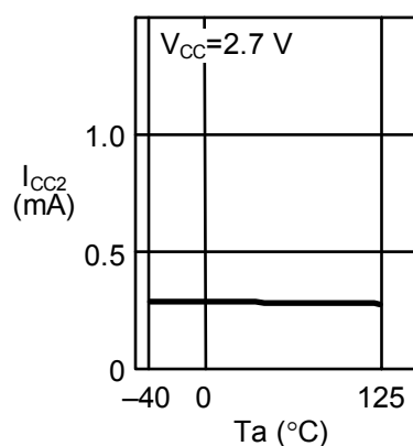
1.9 プログラム時消費電流 I_{CC2} —周囲温度 T_a
