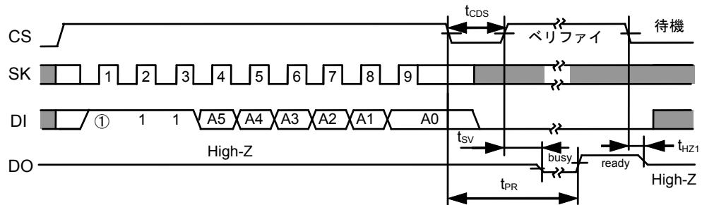
図10 データ消去タイミング (S-93A46A)
