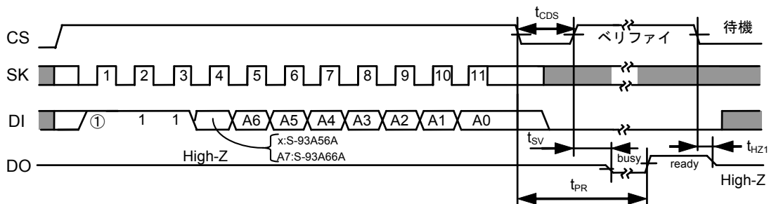
図11 データ消去タイミング (S-93A56A, S-93A66A)
