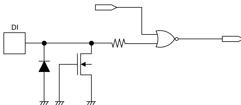
図 23 DI 端子
