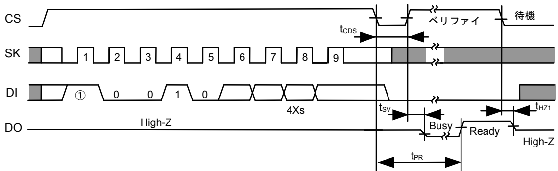
図14 チップ消去タイミング (S-93A46A)
