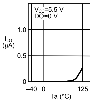
1. 15 出力リーク電流 I_{LO} —周囲温度 T_a
