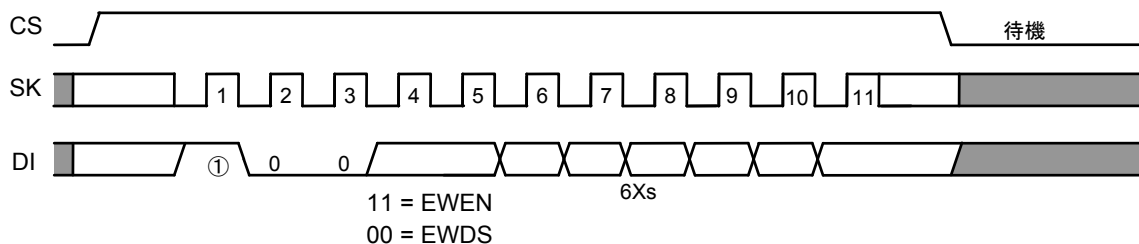
図 17 書き込み許可 / 禁止タイミング (S-93A56A, S-93A66A)
