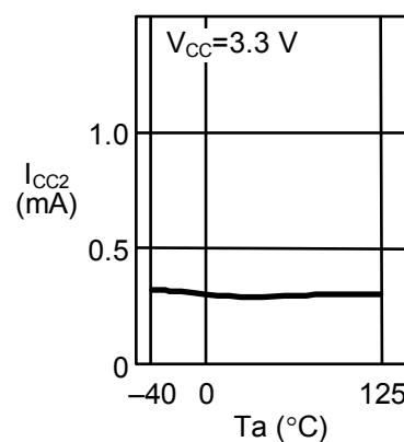
1.8 プログラム時消費電流 I_{CC2} —周囲温度 T_a
