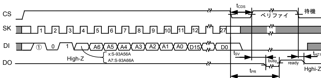
図9 データ書き込みタイミング (S-93A56A, S-93A66A)
