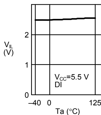
1. 34 低レベル入力電圧 V_{IL} —周囲温度 T_a
