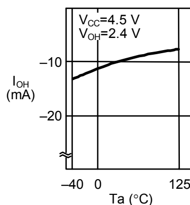
1. 22 高レベル出力電流 I_{OH} —周囲温度 T_a
