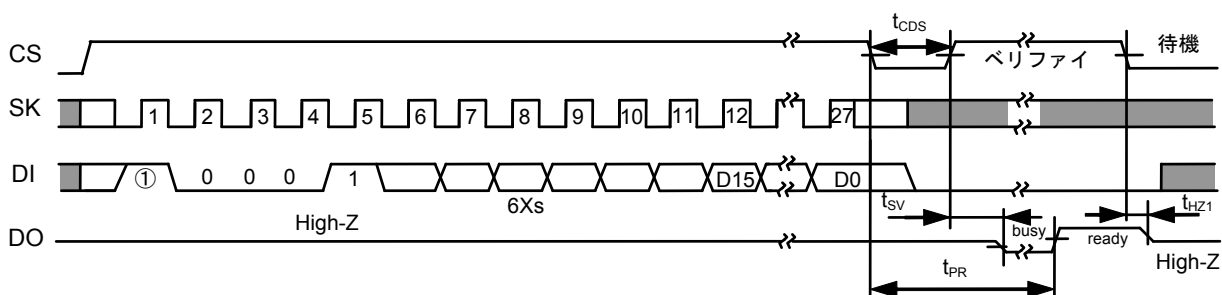
図13 チップ書き込みタイミング (S-93A56A, S-93A66A)
