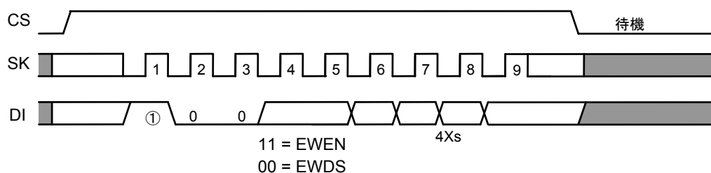
図 16 書き込み許可 / 禁止タイミング (S-93A46A)
