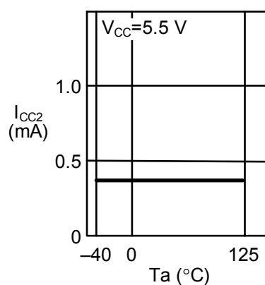
1.7 プログラム時消費電流 I_{CC2} —周囲温度 T_a
