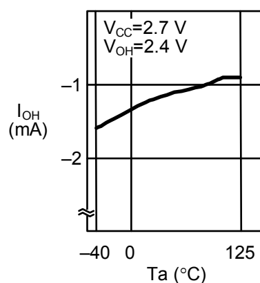
1. 23 高レベル出力電流 I_{OH} —周囲温度 T_a
