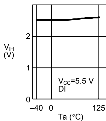
1. 30 高レベル入力電圧 V_{IH} —周囲温度 T_a
