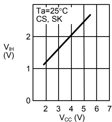
1. 27 高レベル入力電圧 V_{IH} —電源電圧 V_{CC}
