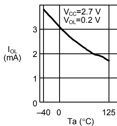
1. 26 低レベル出力電流 I_{OL} —周囲温度 T_a
