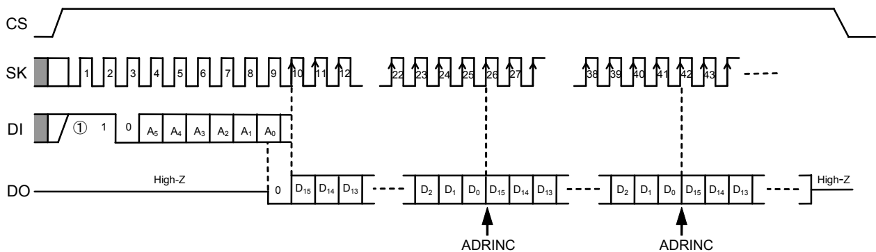
図6 読み出しタイミング (S-93A46A)
