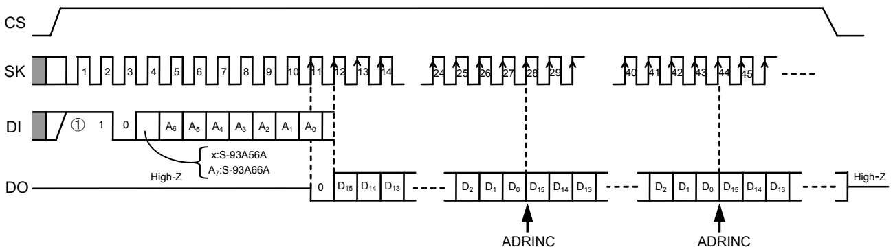
図7 読み出しタイミング (S-93A56A, S-93A66A)
