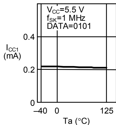
1.1 リード時消費電流 I_{CC1} —周囲温度 T_a
