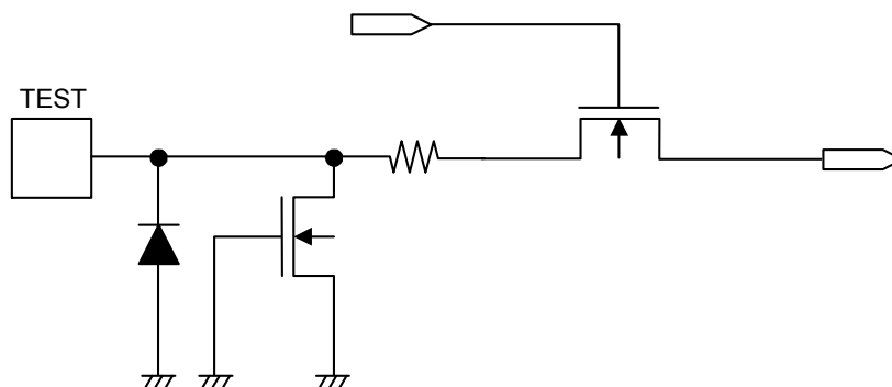
図 24 TEST 端子
