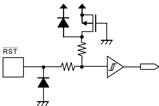
図5 \overline{\text{RST}} 端子
