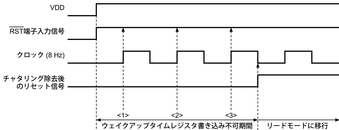
図26 電源投入時のタイミングチャート
