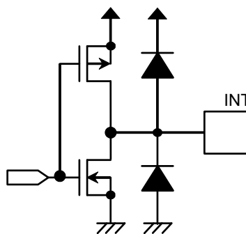
図6 INT端子
