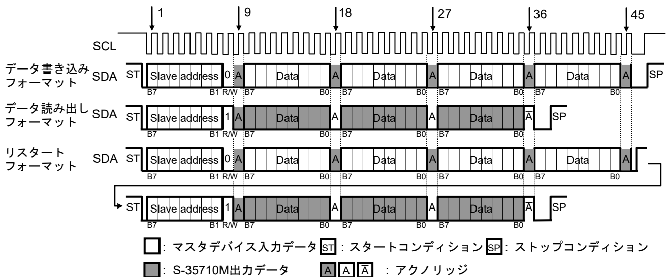
図17 シリアルインタフェースのデータ転送フォーマット
