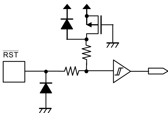
图5 RST端子
