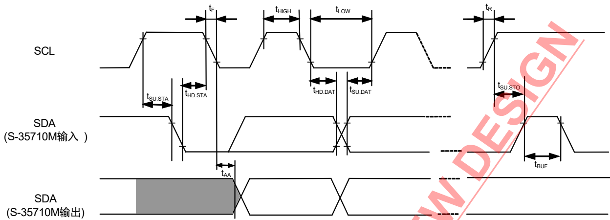
图8 总线时序
