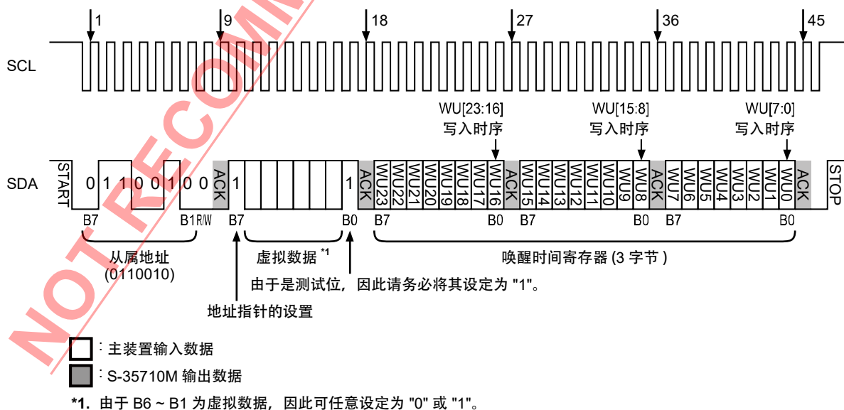
图19 唤醒时间寄存器的写入时序
