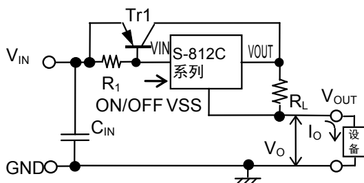
图21 定电流增压电路
