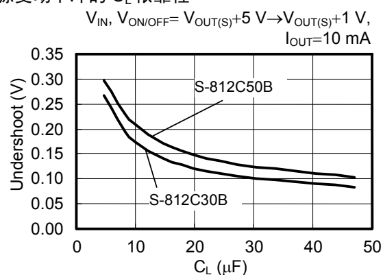
电源变动下冲的 C_L 依赖性
