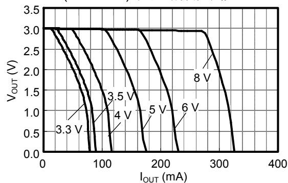
S-812C30A (Ta=25 °C) 无短路保护功能
