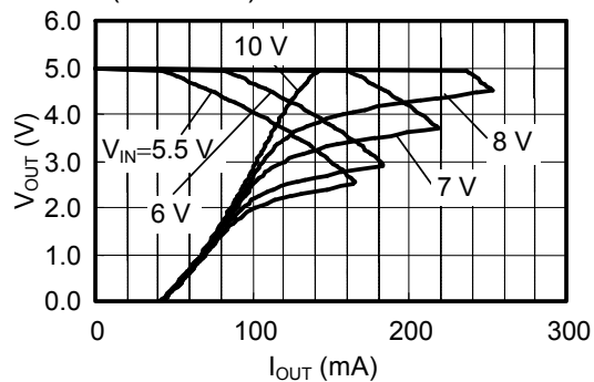
S-812C20A (Ta=25 °C) 无短路保护功能
