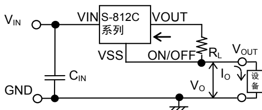
图20 定电流电路
