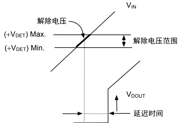
图30 解除电压
