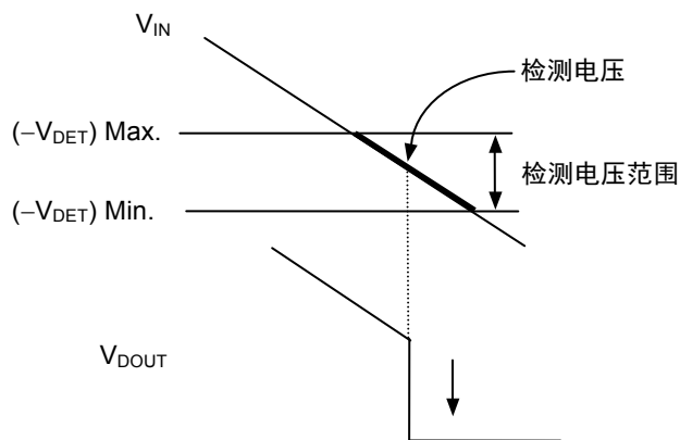
图29 检测电压
