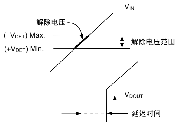
图30 解除电压
