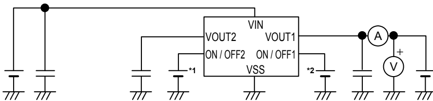
图13 测定电路3
