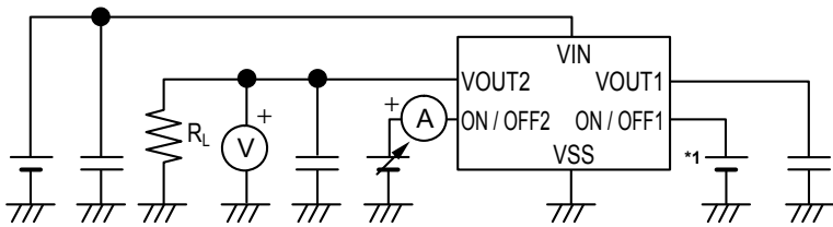
图16 测定电路6
