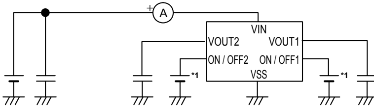
图12 测定电路2
