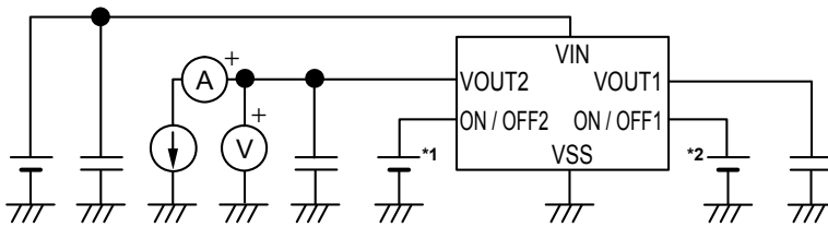
图11 测定电路1
